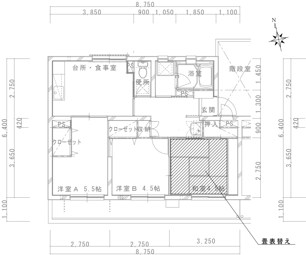
1号棟 平面図 S=1/100
