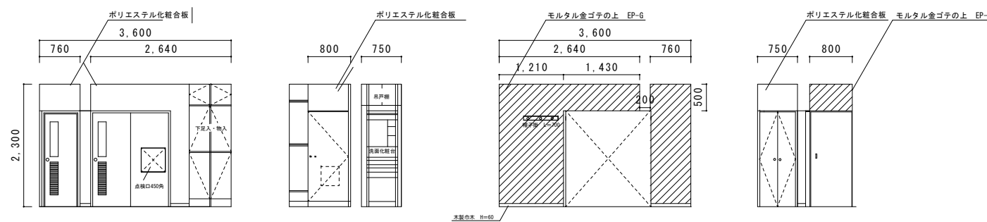
玄関・ホール壁展開図 S=1/100
