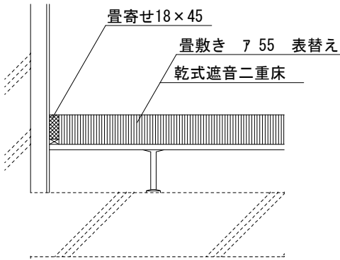
和室床断面図 S=1/10
