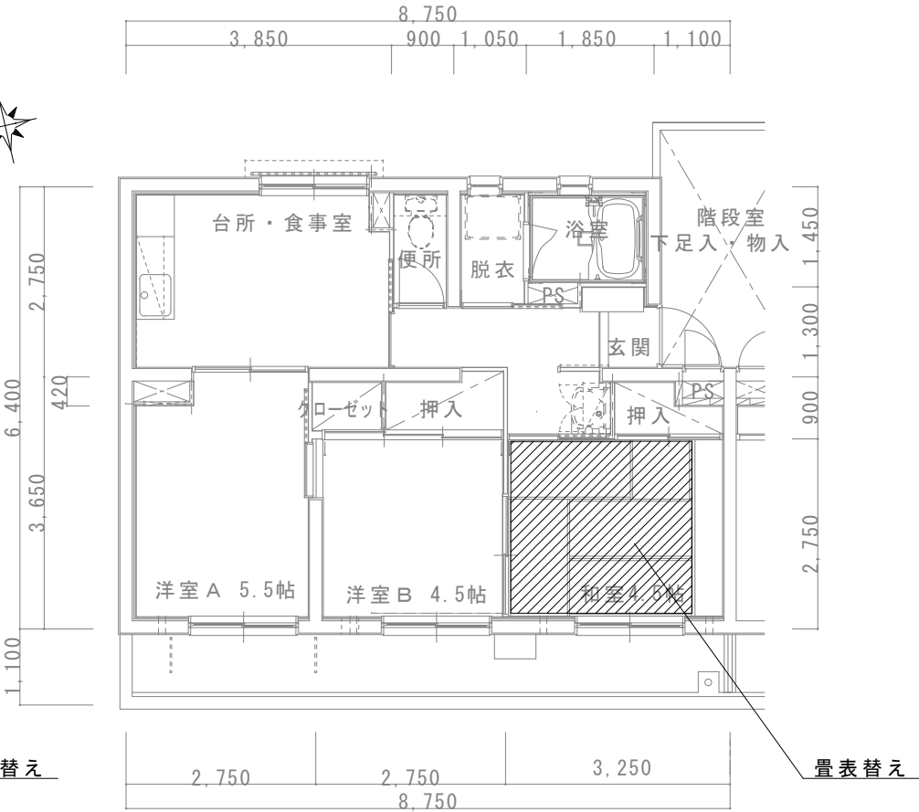
2号棟 平面図 S=1/100
