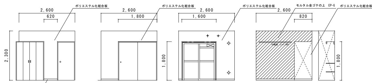
洋室 B 壁展開図 S=1/100
