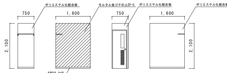
便所壁展開図 S=1/100
