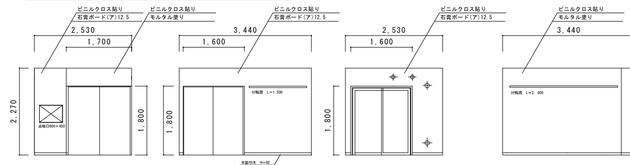
台所・食事室壁展開図 S=1/100
