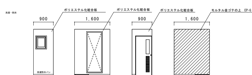
洗濯室壁展開図 S=1/100
