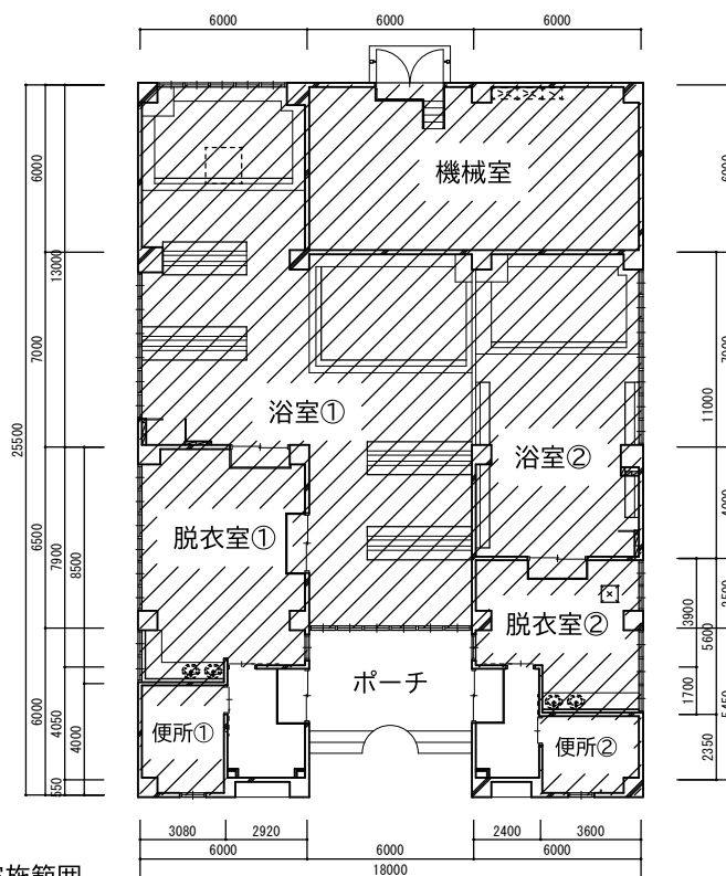
81号 平面図 S=1/300
