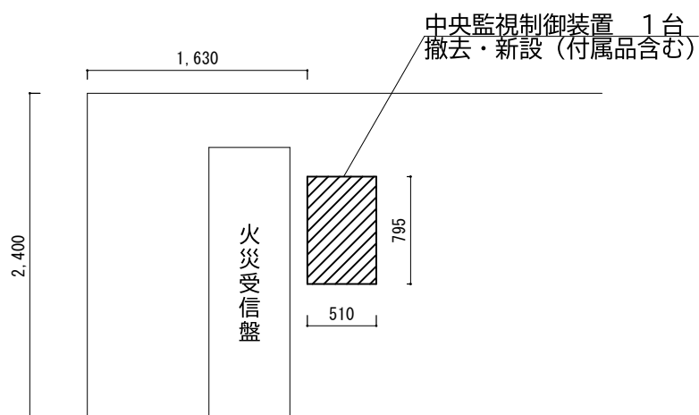
当直室（西側）立面図 S=1/X
