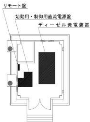
図2.1-平面図（非常用発電機室）
