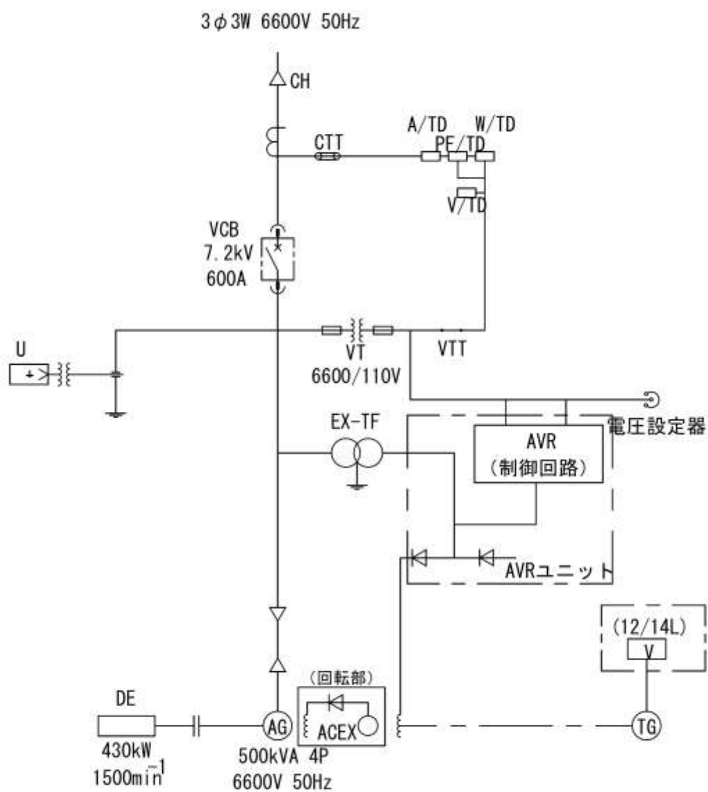
図3-単線結線図
