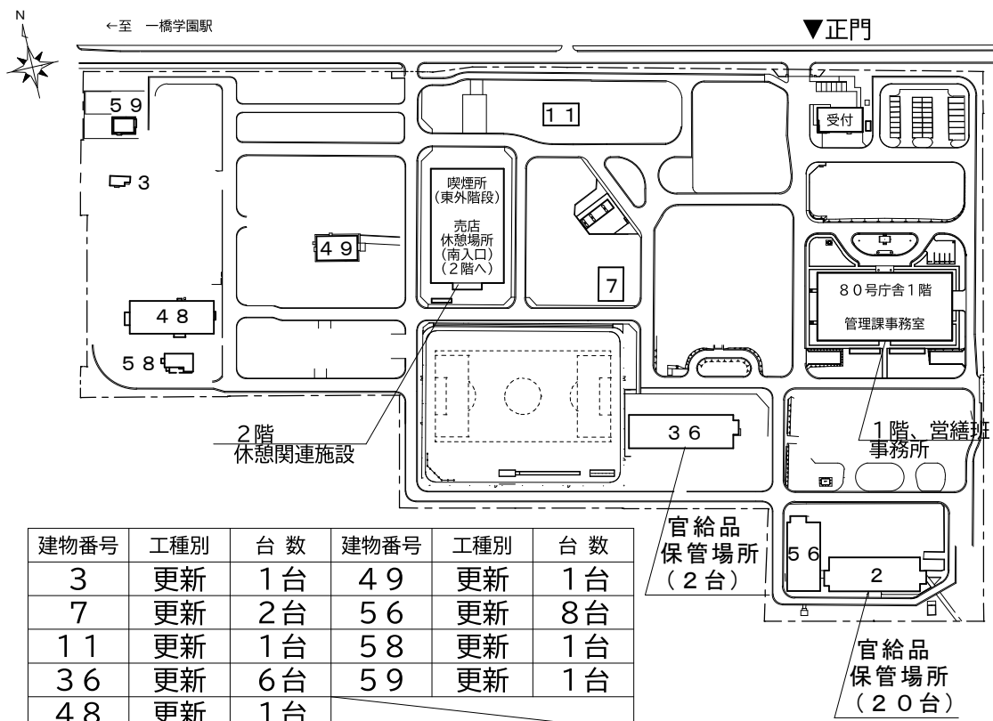
配置図 S=1/X
