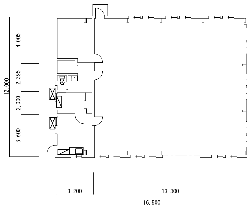
7号建物 空調機設置位置図 S=1/X
