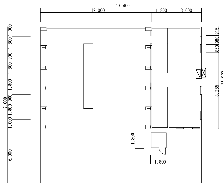
11号建物 空調機設置位置図 S=1/X
