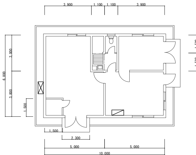
5 9号建物 空調機設置位置図 S=1/X
