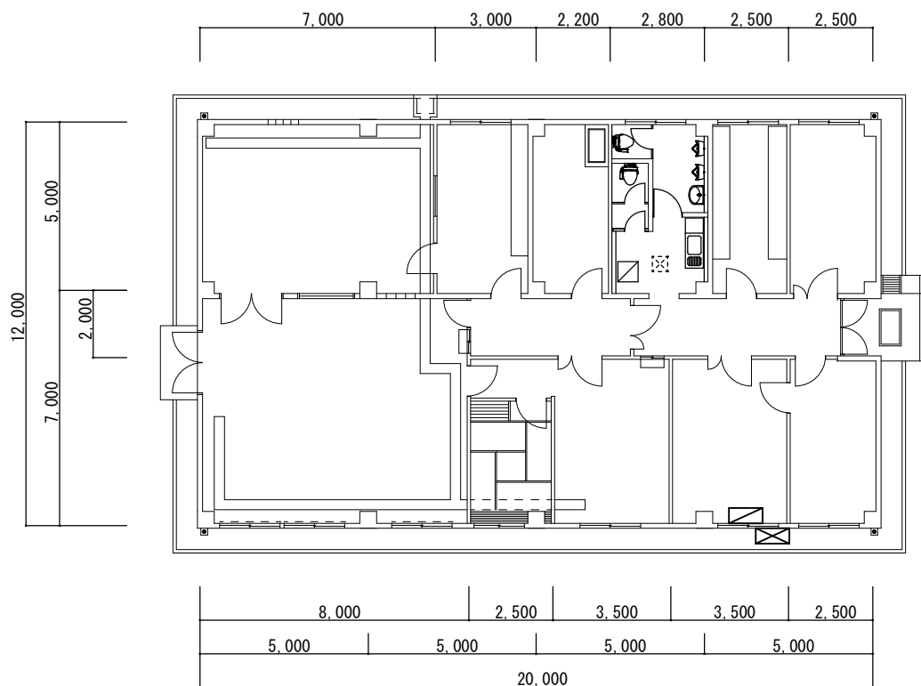
49号建物 空調機設置位置図 S=1/X
