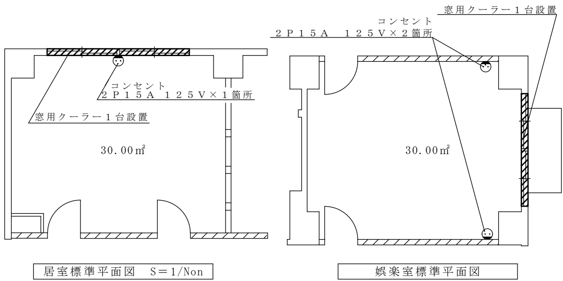
64号建物設置標準図 S=1/X
