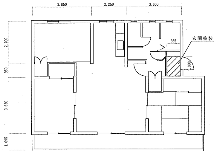
第3宿舍1号棟204号室平面图
