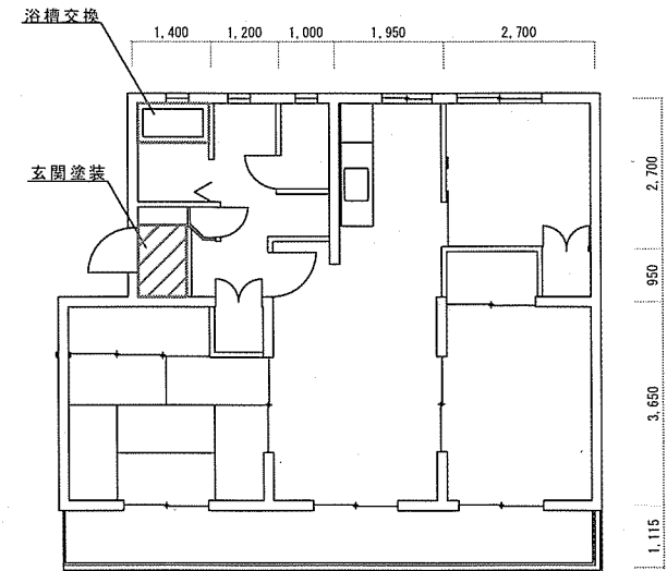
第3宿舍2号棟201号室平面图
