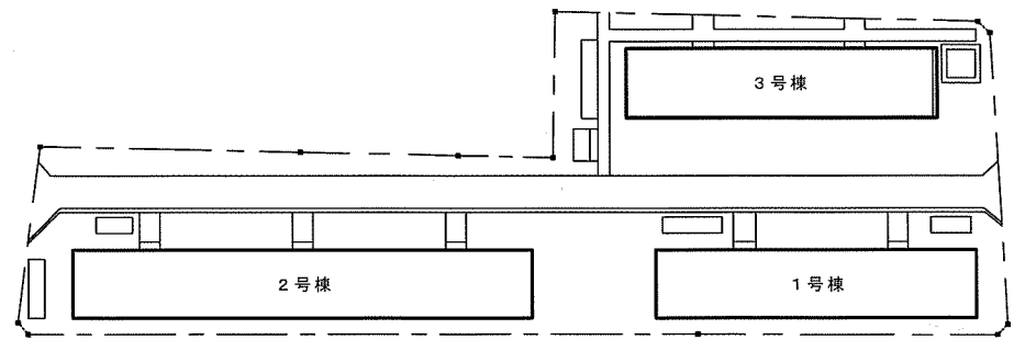
第3宿舎配置図 S=1:700
