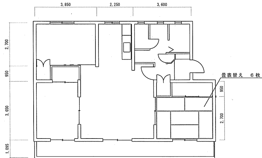
第3宿舍1号棟304号室平面图
