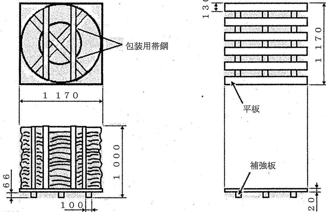
図5-包装要領
