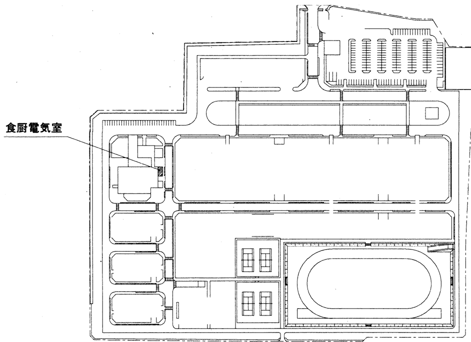
配置図 S=1/4000
