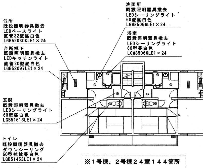
宿舎居室照明器具配置図 S=1/150
