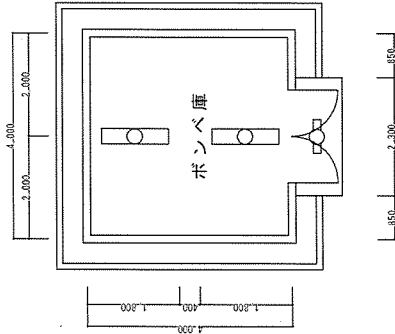
305号ポンベ庫平面図 S=1:100
