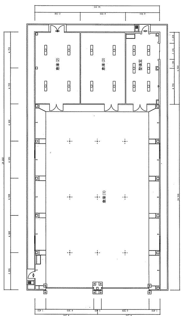
311号倉庫平面図 S=1:200
