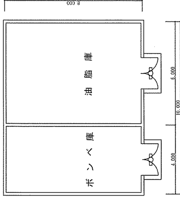
307号ポンベ庫・油脂庫平面図 S=1:100
