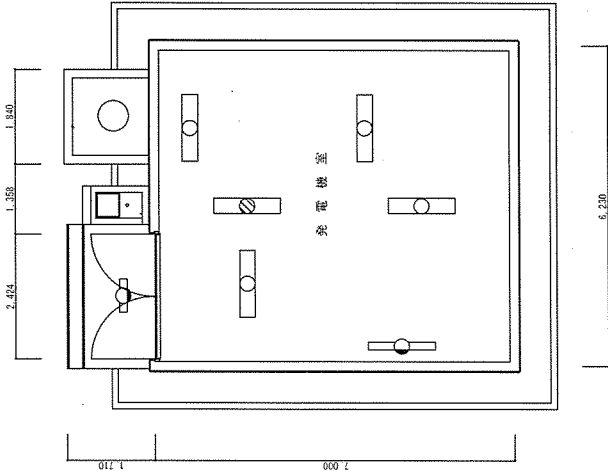
319号発電機室平面図 S=1:100
