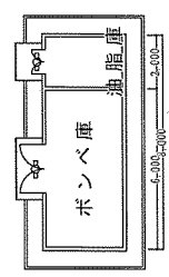
312号ボンベン庫・油脂庫平面図 S=1:200
