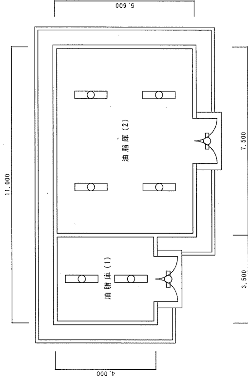
304号油脂庫平面図 S=1:100
