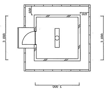
47号倉庫平面図 S=1:100
