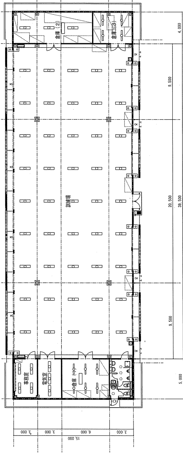
320号訓練施設平面図 S=1:200
