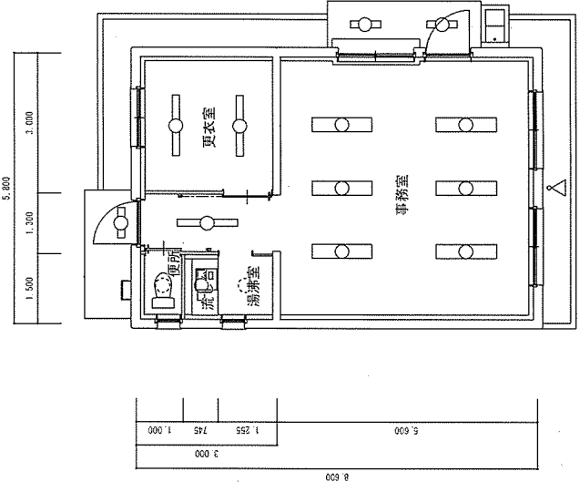
318号給油所平面図 S=1:100
