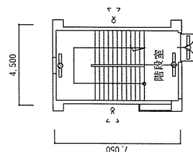
3324号訓練施設塔屋平面図 S=1:200
