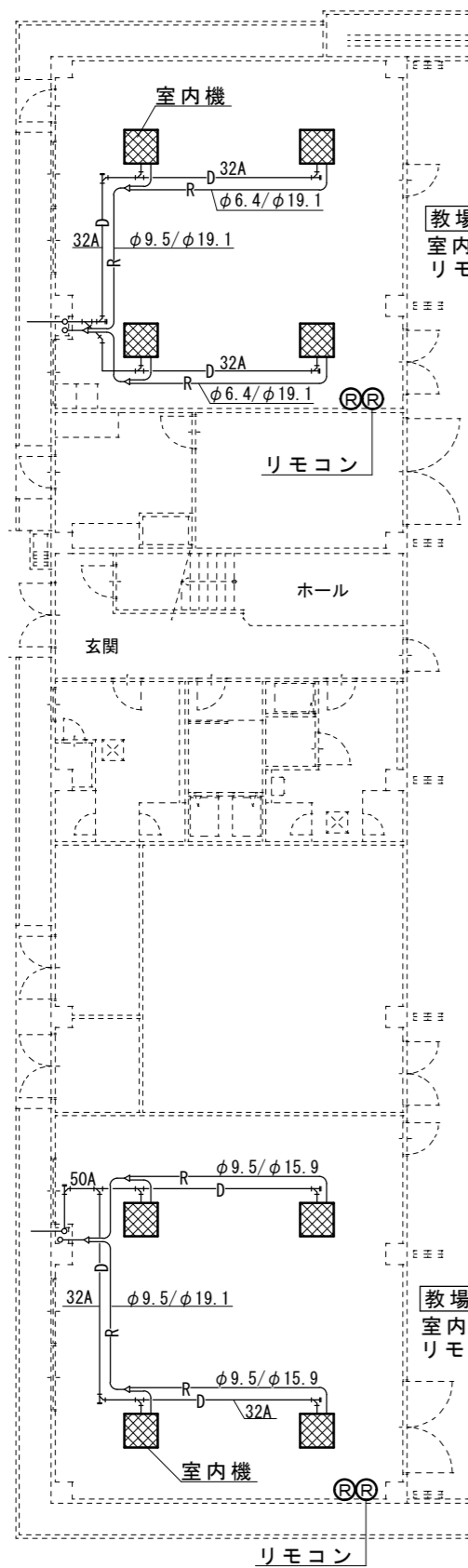
1階平面図 S=1/200
