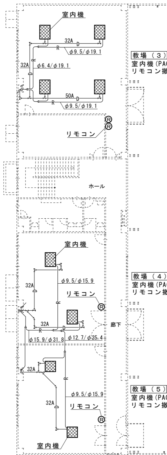
2階平面図 S=1/200
