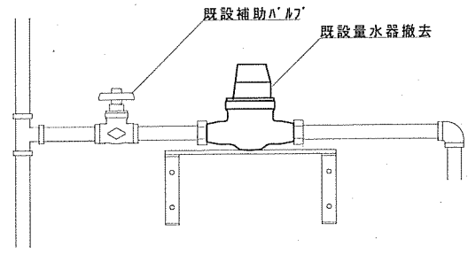
改修前標準配管図 S=1:X
