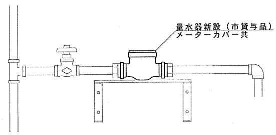
改修後標準配管図 S=1:X
