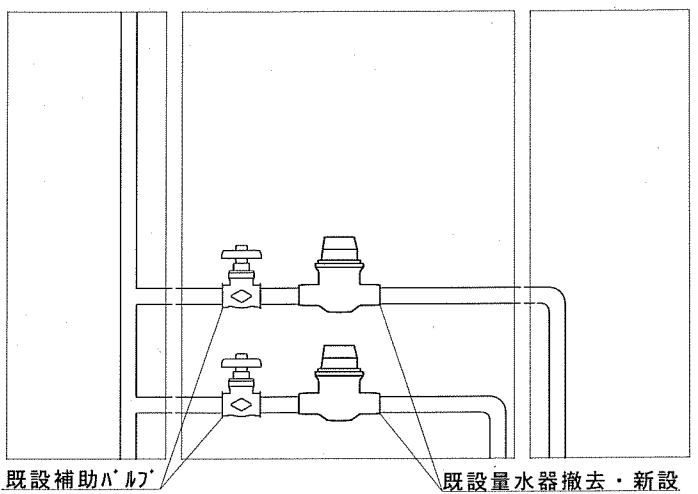
既設P.S内標準姿図 S=1:X
