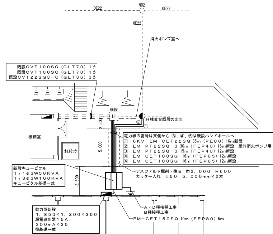
補修後梨ヶ原廠舎電力配線図 S = 1 : X
