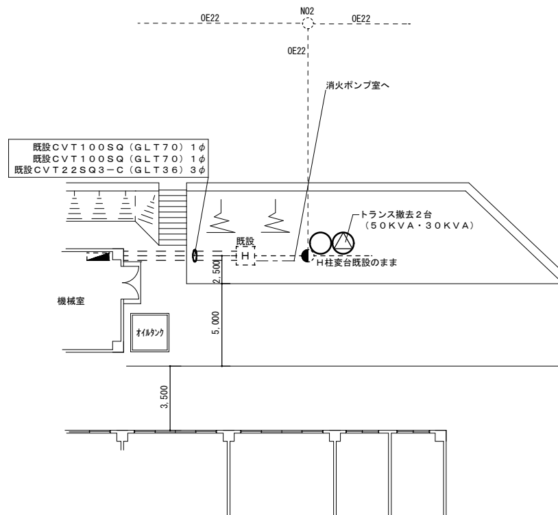
補修前梨ヶ原廠舎電力配線図 S = 1 : X
