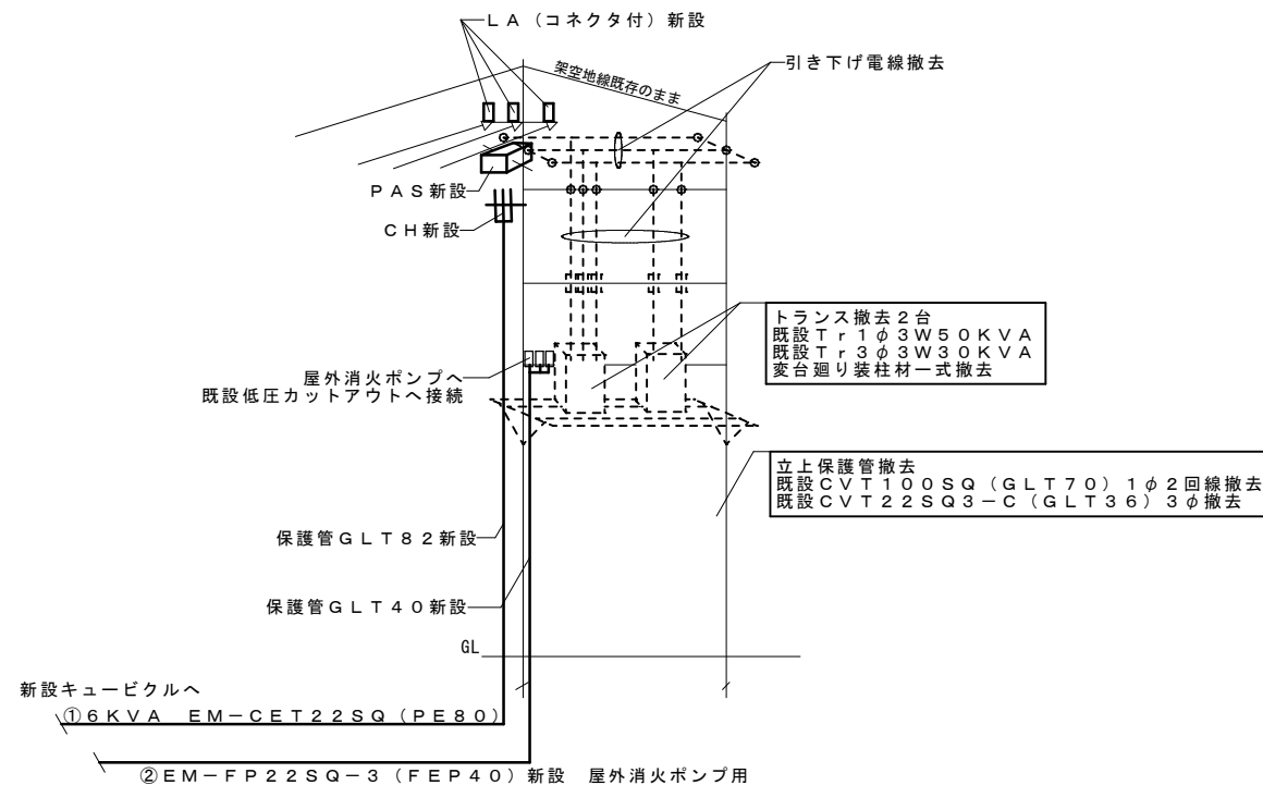
補修梨ヶ原廠舎H変台装柱図 S = 1 : X
