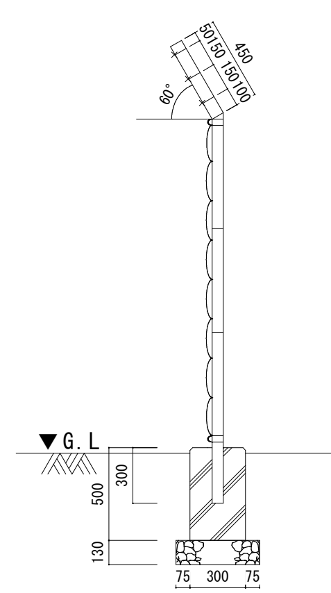
既設万年塀（撤去）詳細図 S=1/Non
