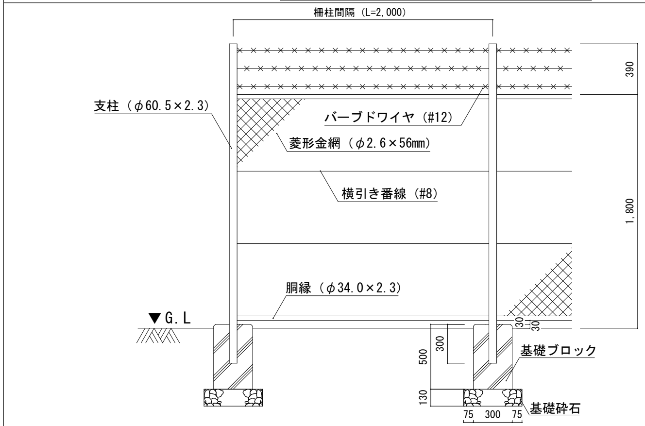
新設外柵詳細図 S=1/Non
