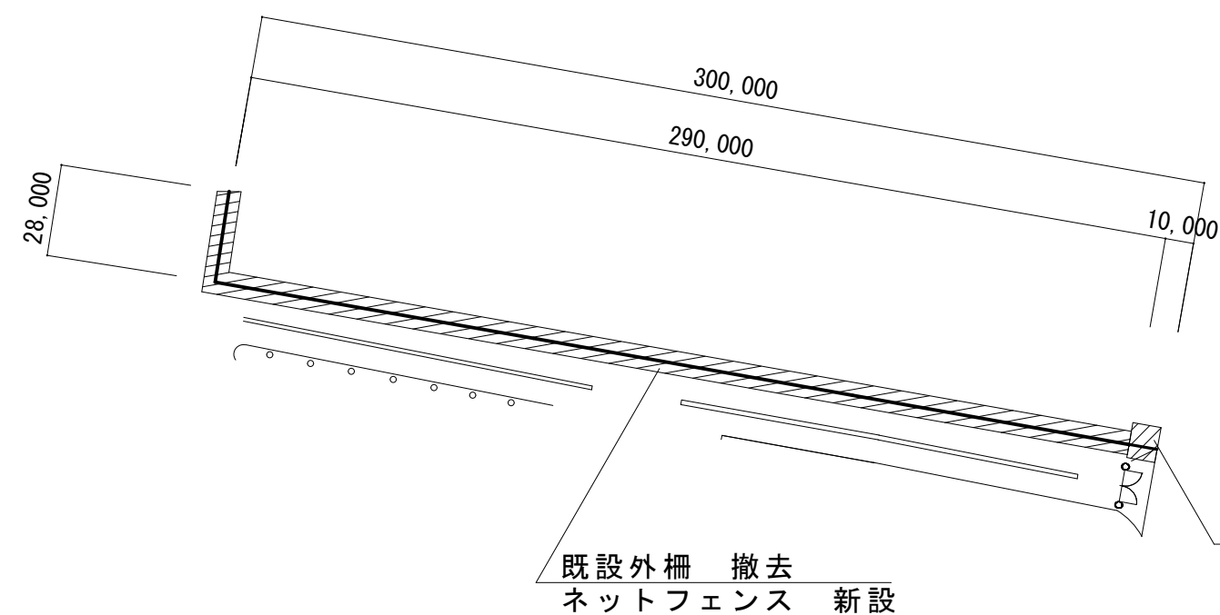
詳細配置図 S=1/Non
