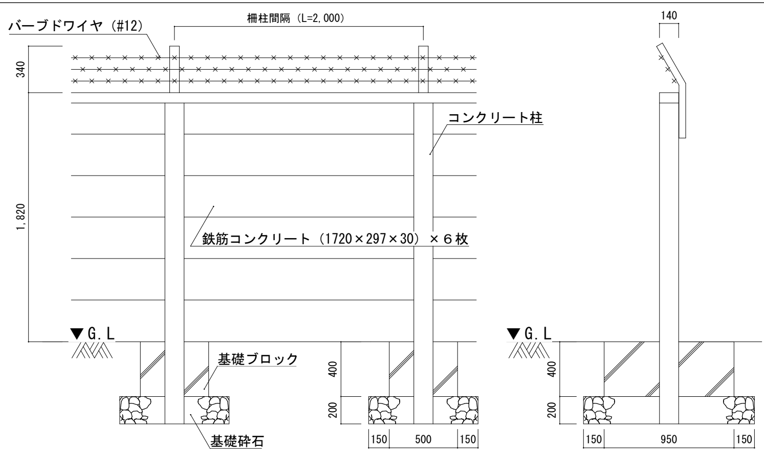
既設万年塀（撤去）詳細図 S=1/Non
