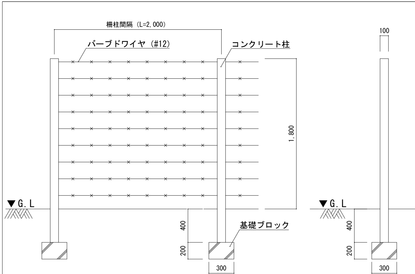
既設外柵（撤去）詳細図 S=1/Non
