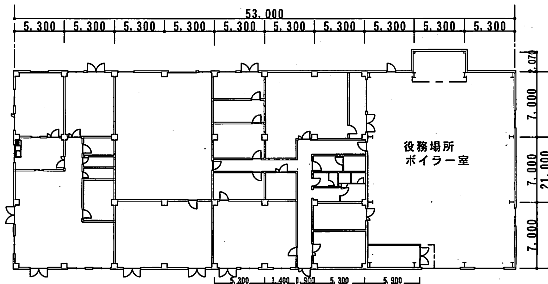
設備管理棟平面図 S = 1 : 400
