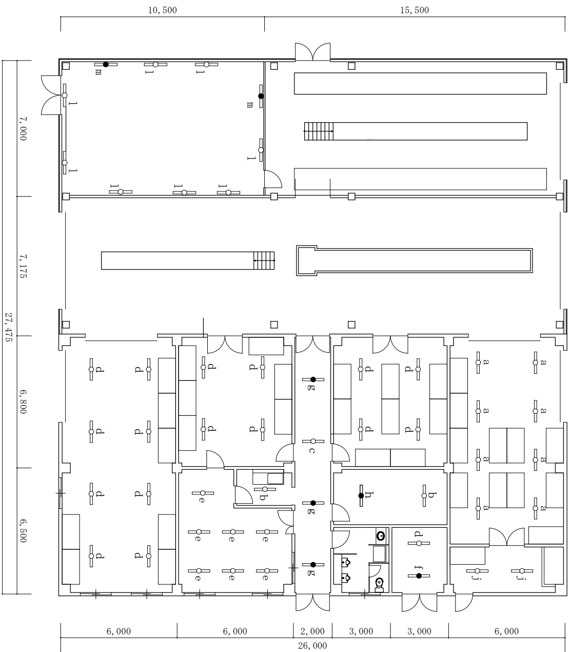
1 2 6 号改修後 平面図 S=1:200
