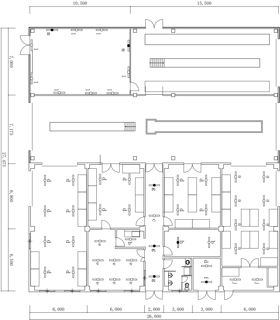
1 2 6号改修前 平面図 S=1:200
