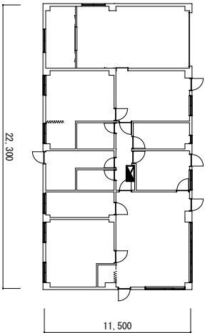
163号警衛所平面図 1：300
