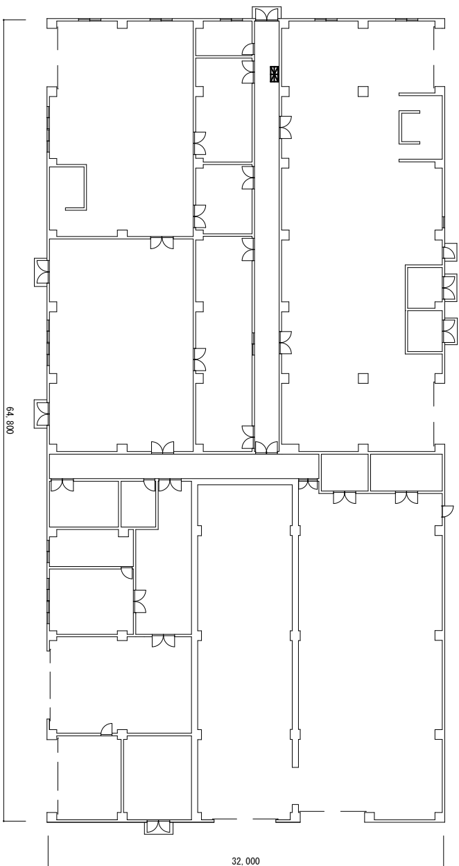
120号SSM試験場平面図 1：300
