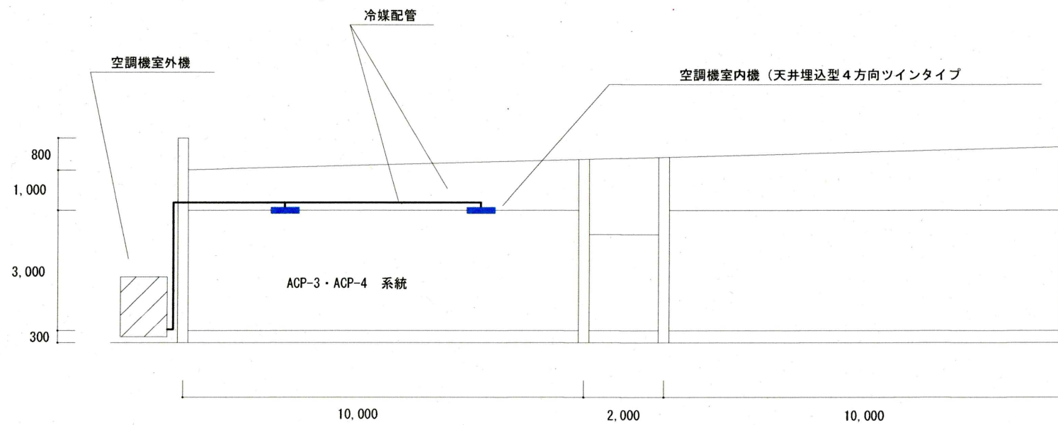
建物断面図 1 : X
