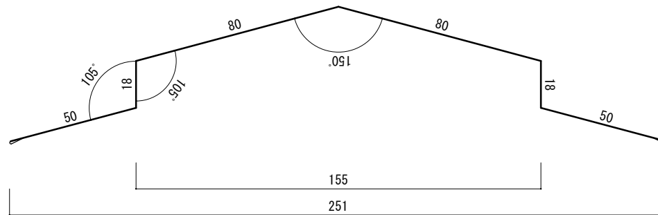
棟板断面図 S=1/2
