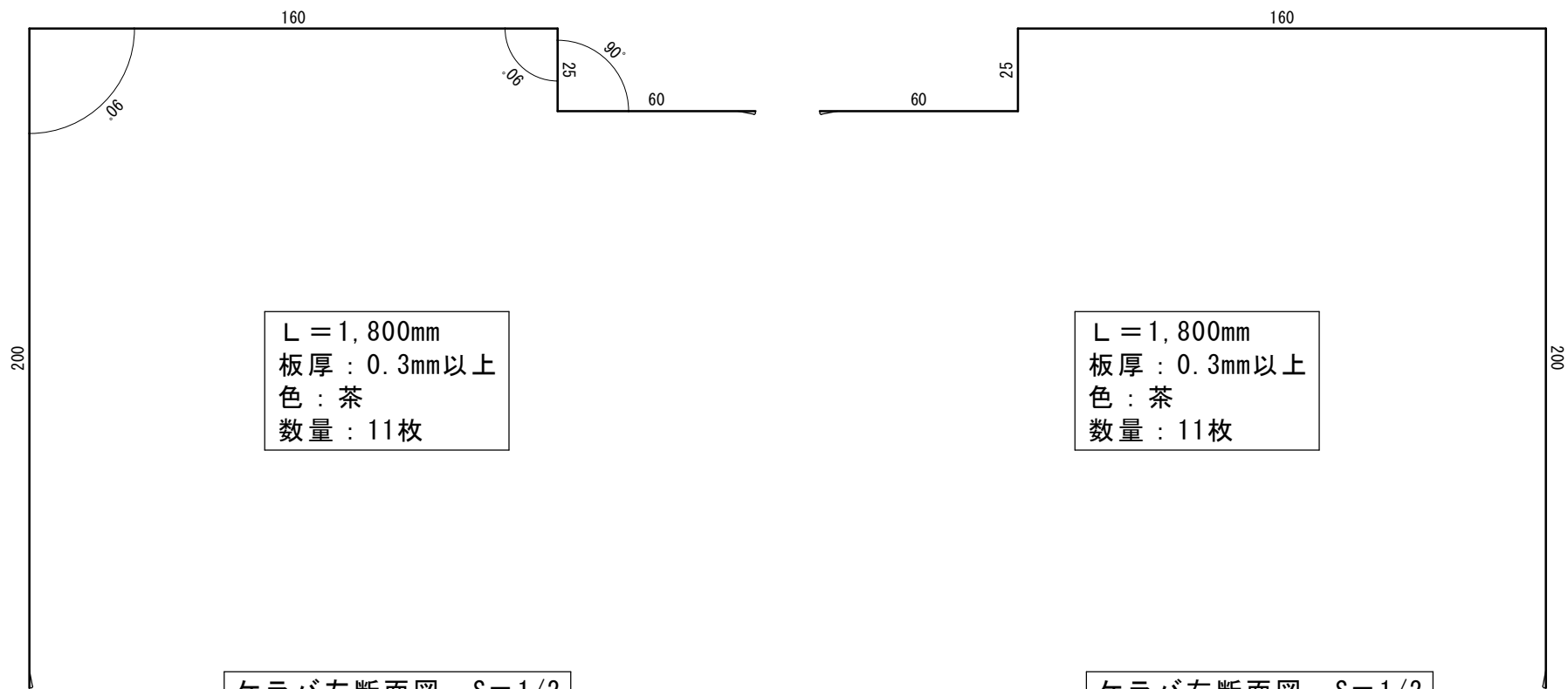
ケラバ左断面図 S=1/2
