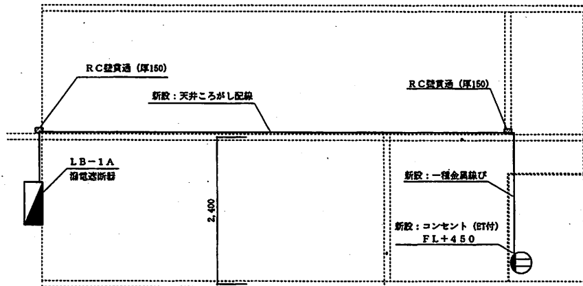
断面図 1/X
