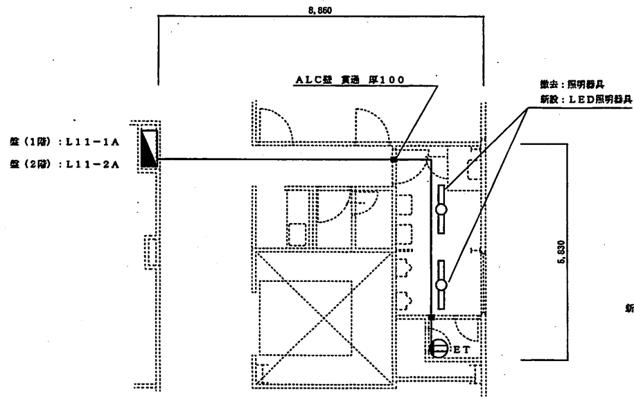
平面図 S=1/100
