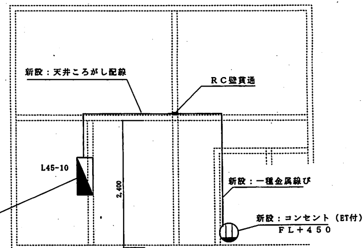
断面図 1/50
