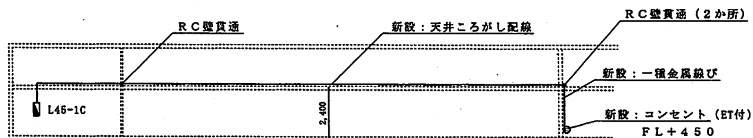
断面図 1/200
