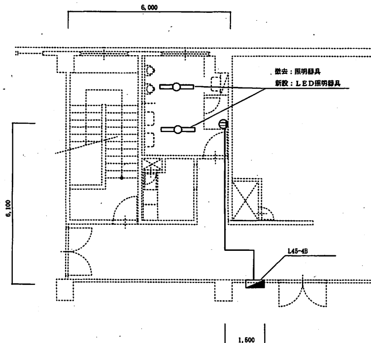
平面図 1/100
