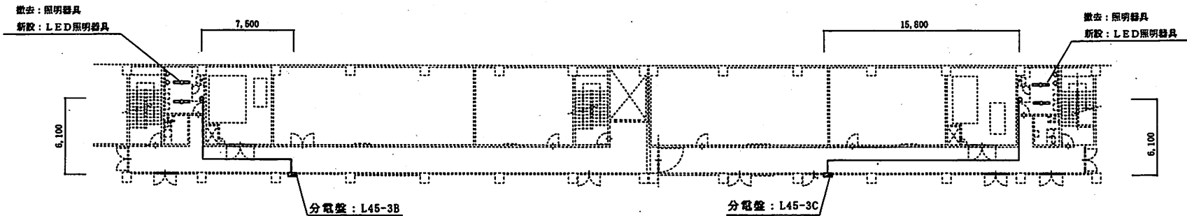
平面図 1/300
