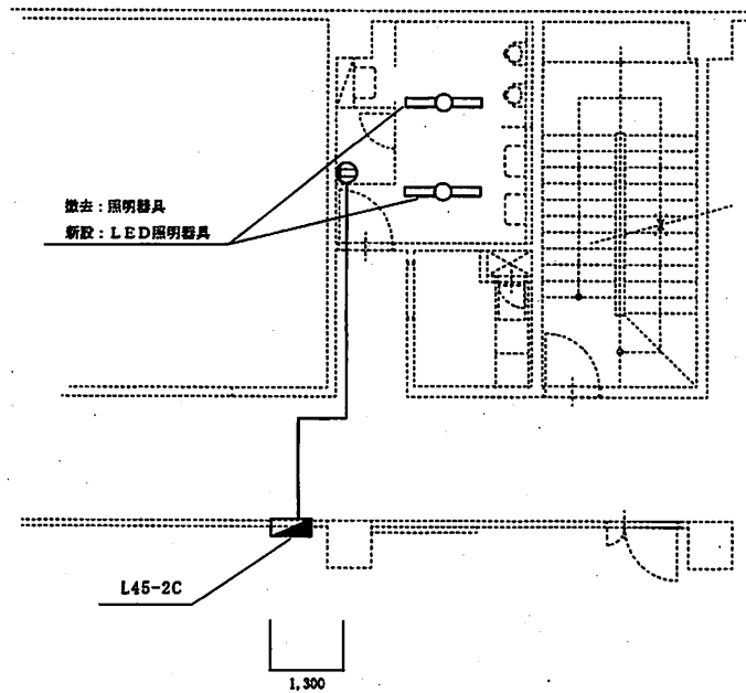
平面図 1/100
