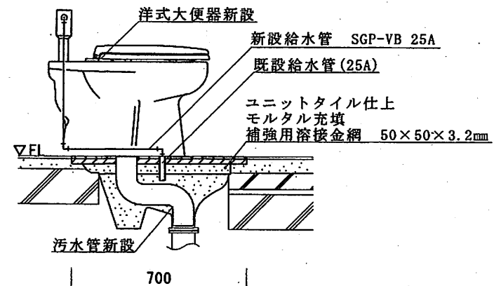
施工後断面
