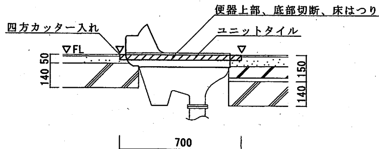
施工前断面
