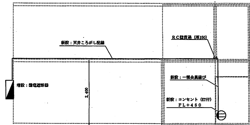
断面図 1/X
