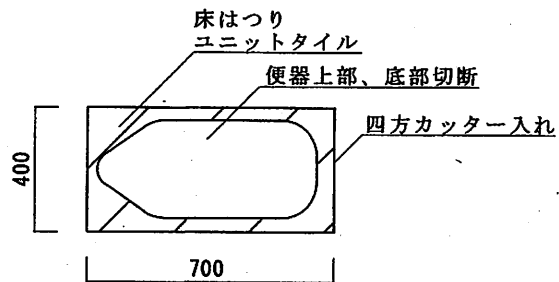
施工前平面
