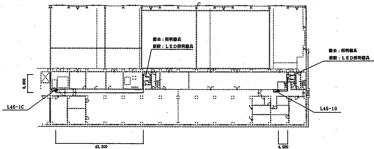
平面図 1/X
