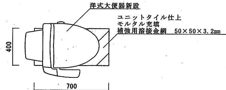
施工後平面
