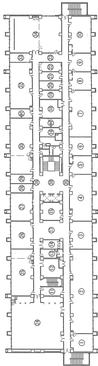
155号建物R F平面図 S=1/500
