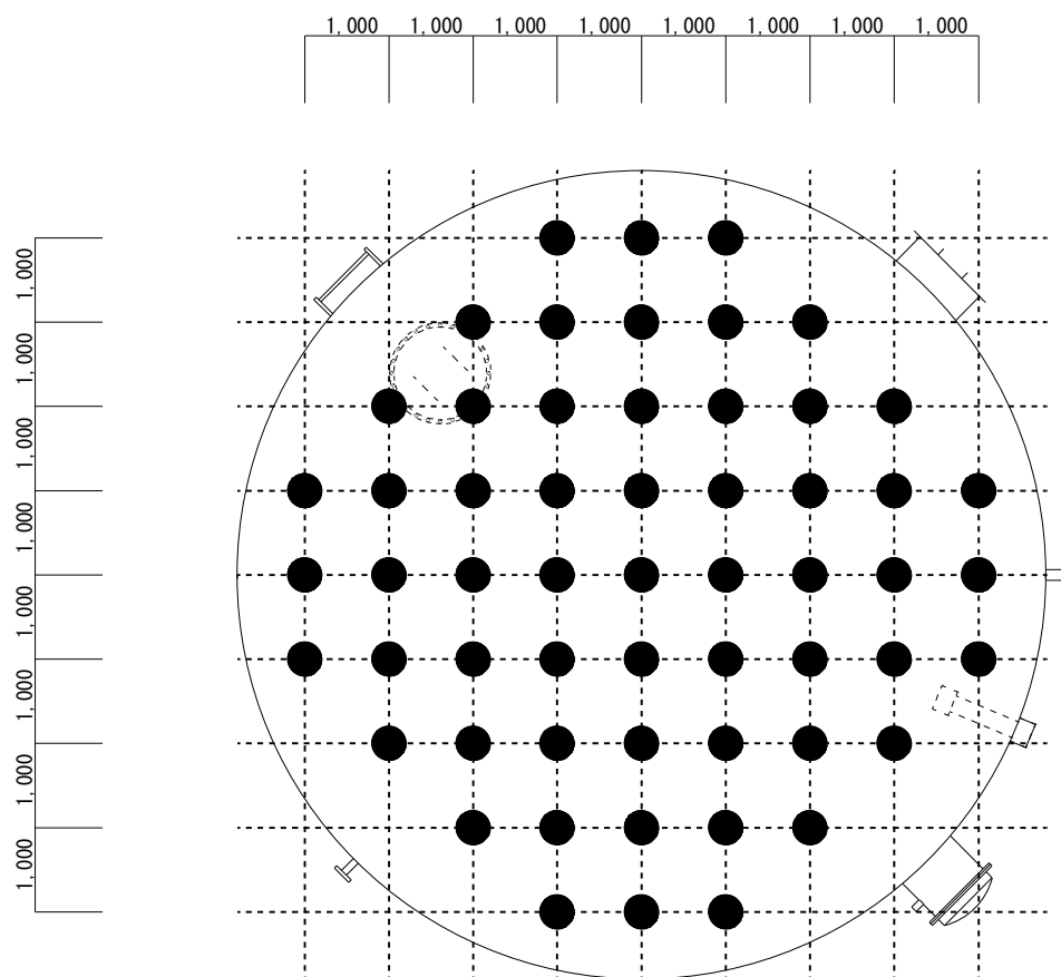
燃料タンク平面図 1:50
