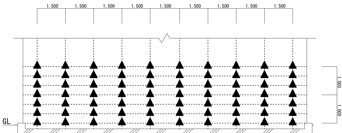
燃料タンク展開図 1:X
