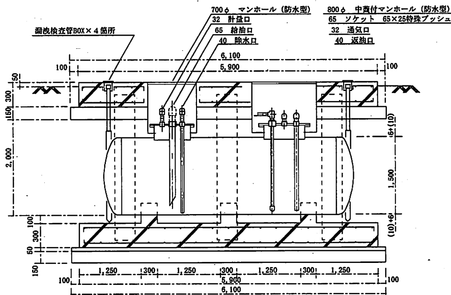
303号建物 地下タンク詳細図 S=1/X
