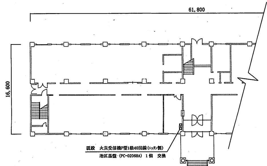
301号建物1階 平面図 S=1/X
