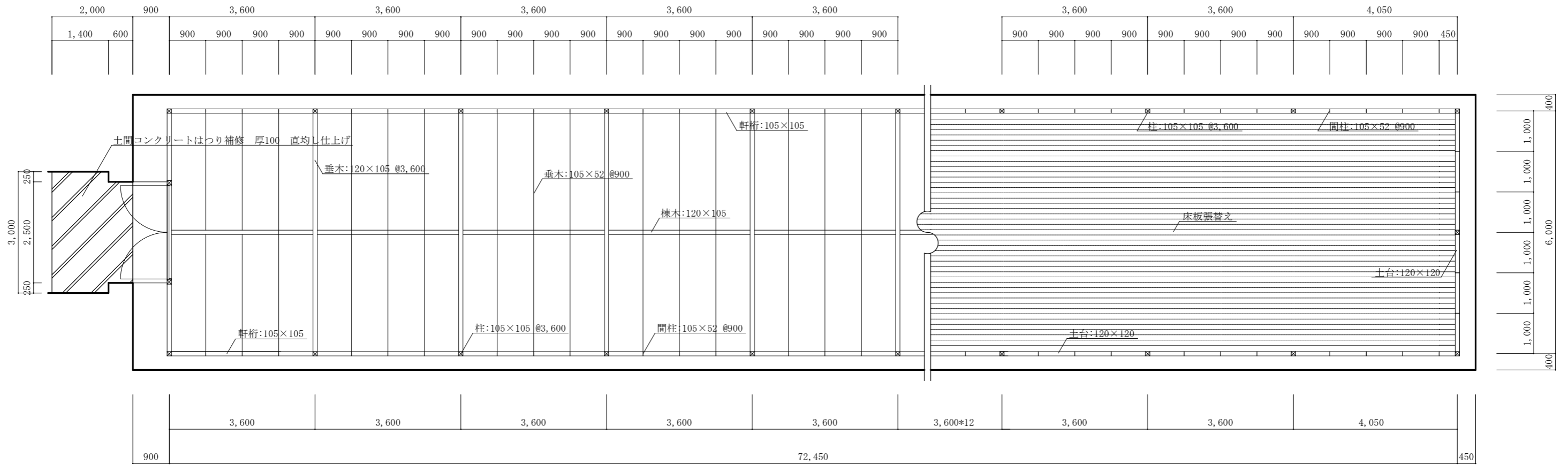
内構詳細平面図 S=1:100
