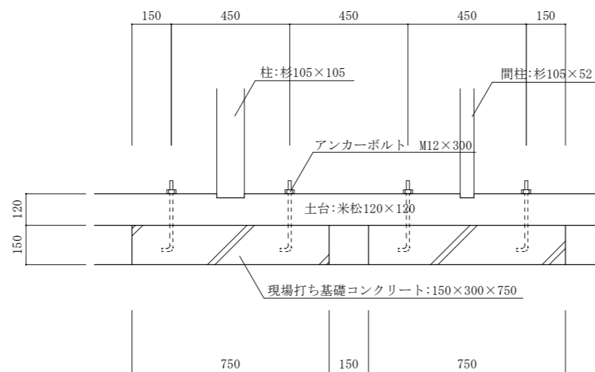
軒側現場打ち基礎コンクリート部詳細図 S=1:20
