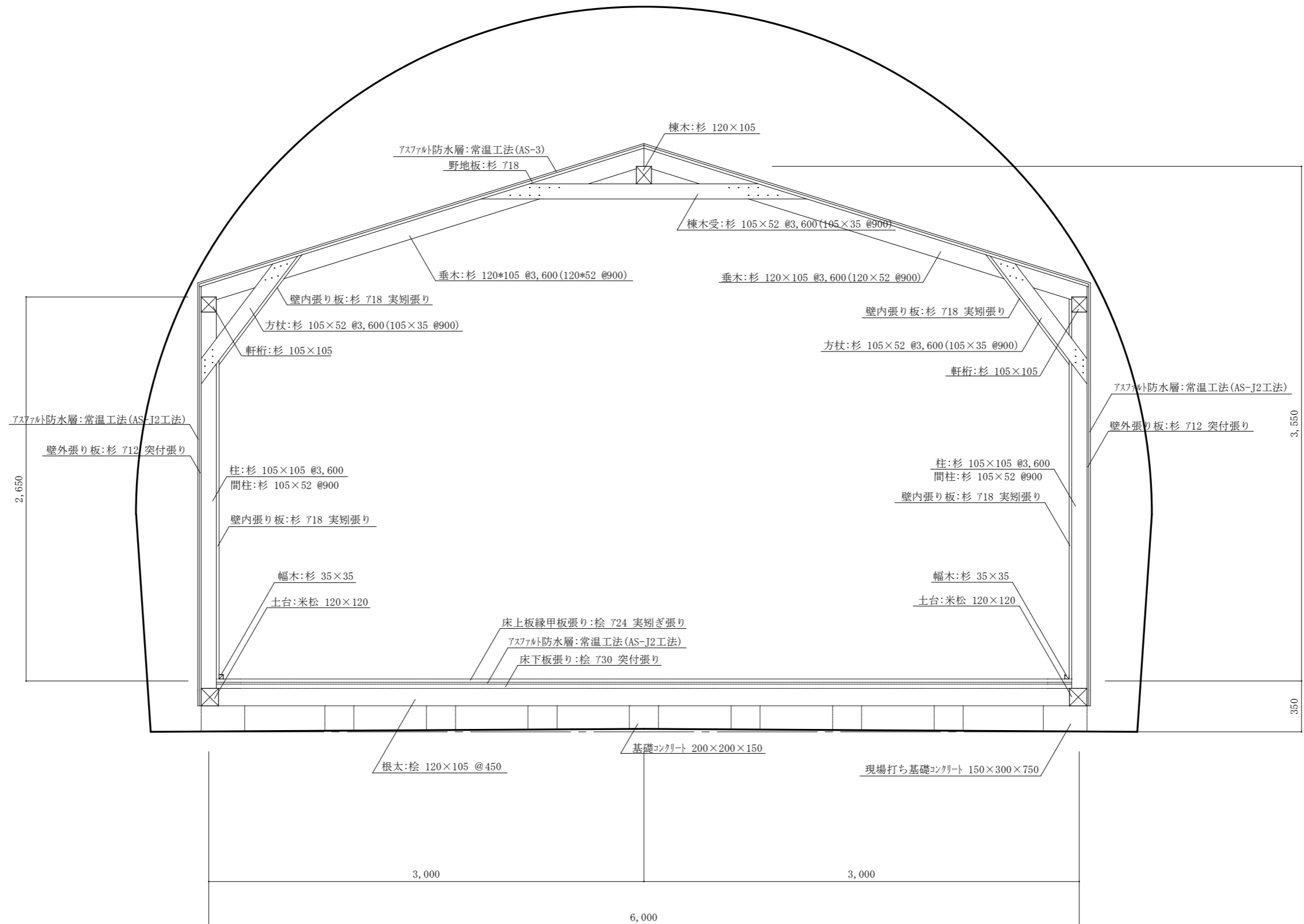
補修後 A - A 断面図 S=1:30
