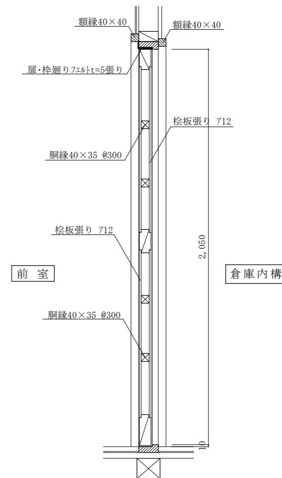
断面図 S=1:20
