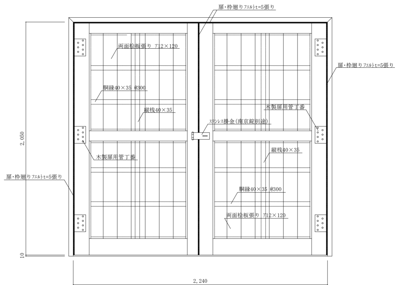
前室側姿図 S=1:20
