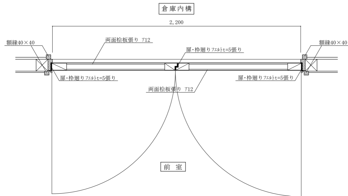
平面図 S=1:20
