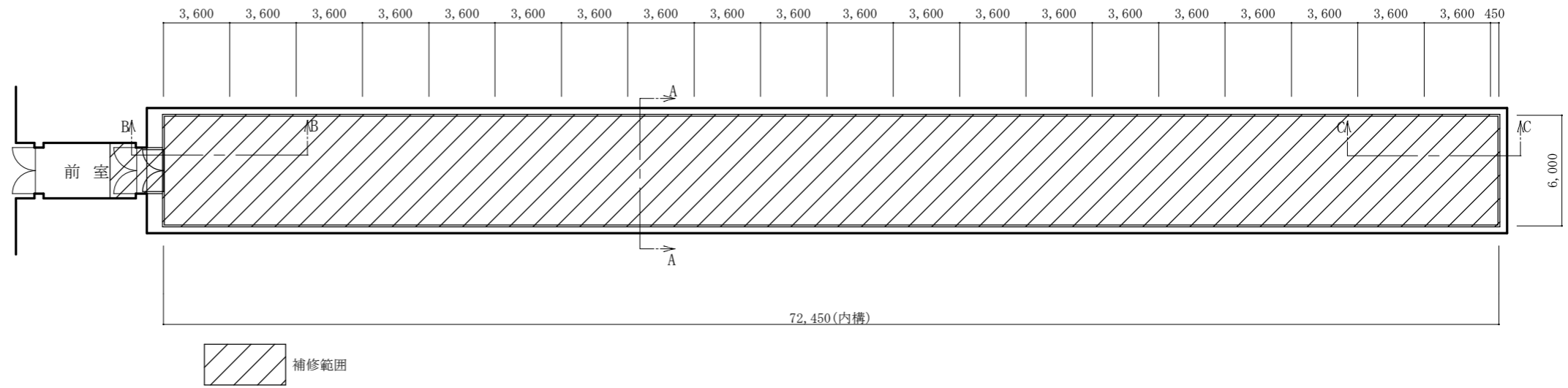
内構平面図 S=1:300
