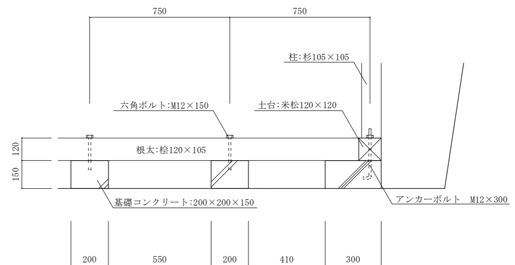
基礎コンクリート部詳細図 S=1:20
