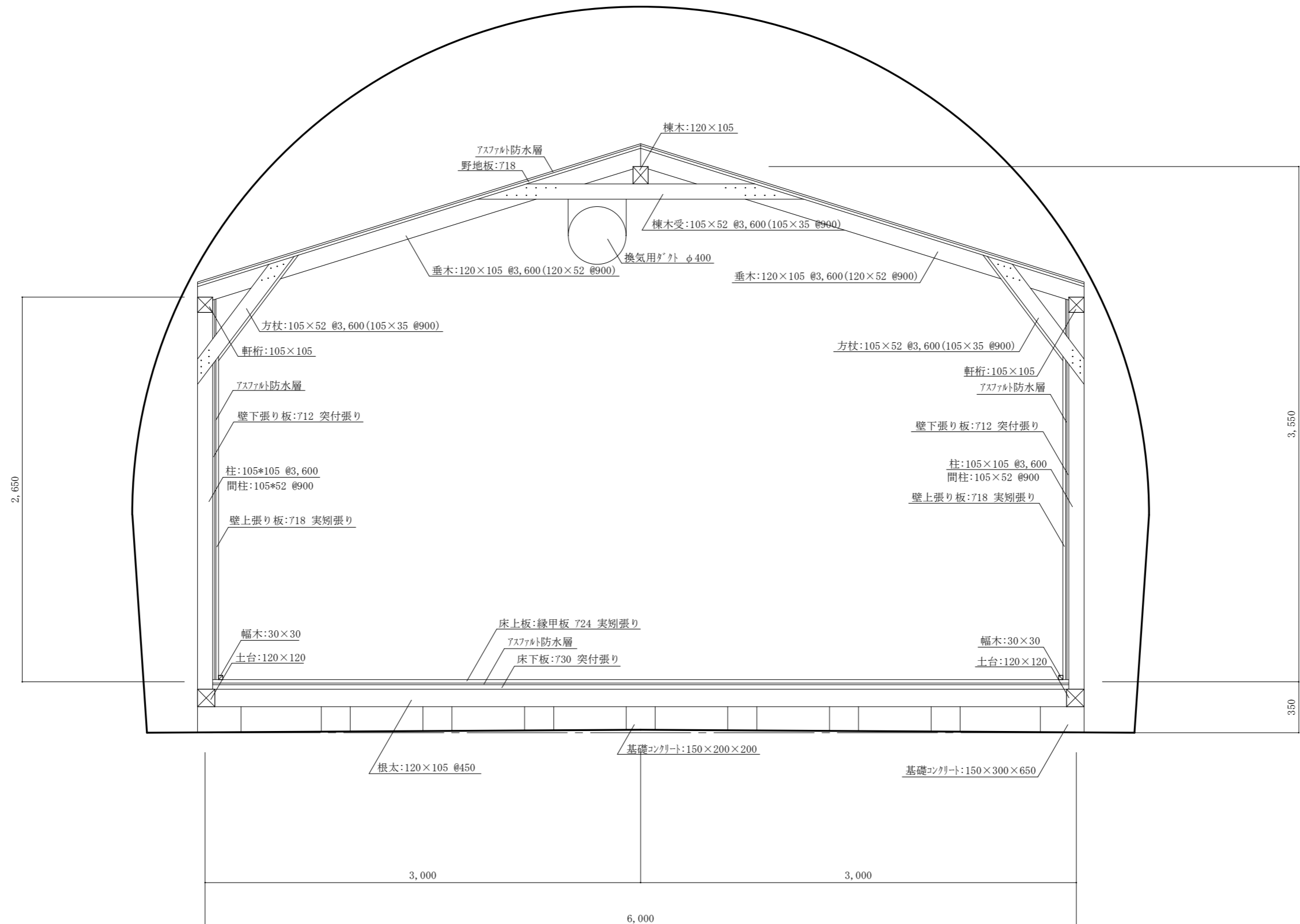
補修前 A - A 横断面図 S=1:30
