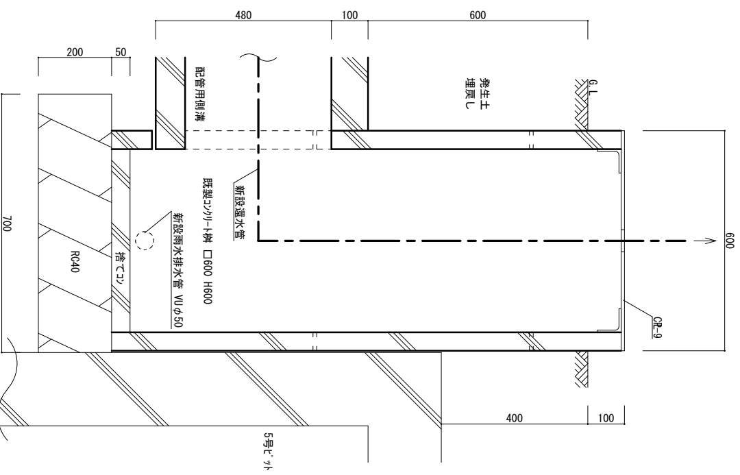
新設接続桝④詳細図 S=1/10
