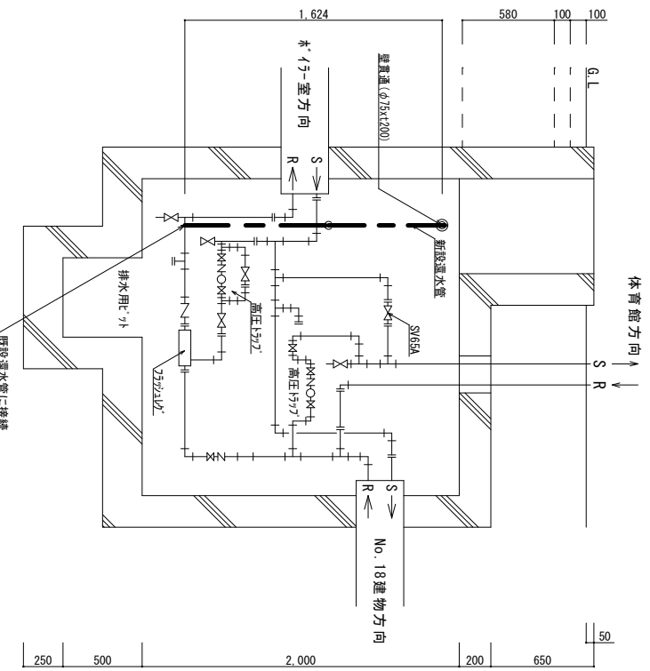
既設蒸気管用「B-B」断面図 S=1:30
