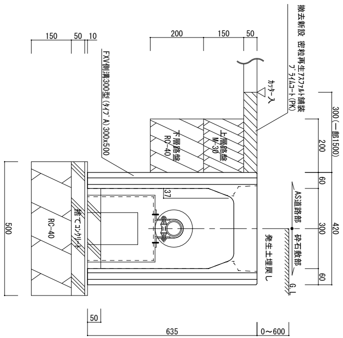
新設配管用U型側溝詳細図 S=1/10
