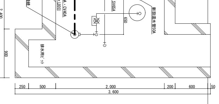
「A-A」断面図 S=1:30
