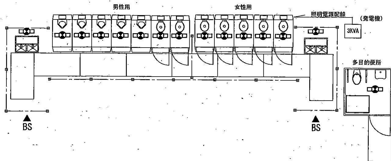
①設置標準図(第1駐輪場) S=1/100
