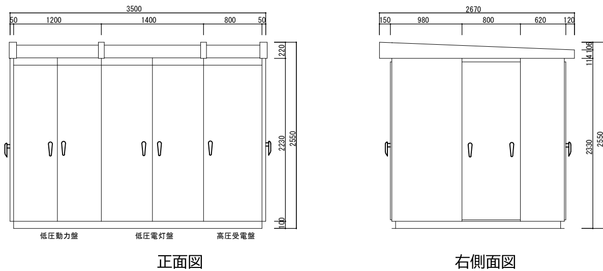
図6.2-キュービクル姿図 (No.9)
