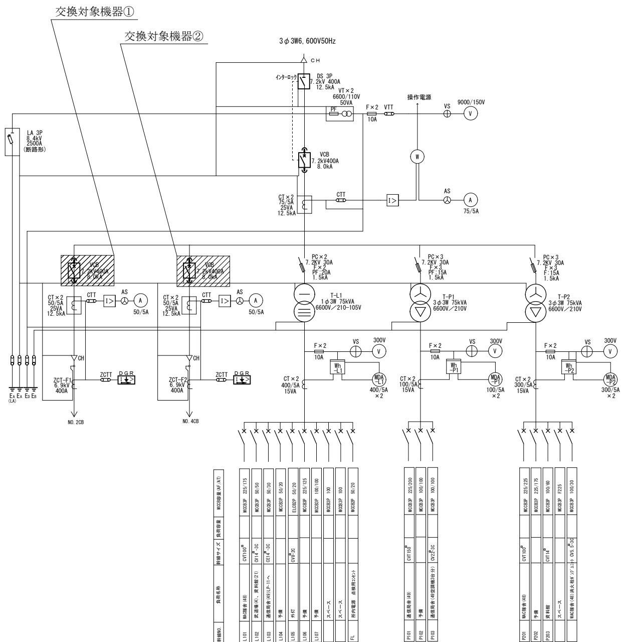
図2.1-単線結線図 (No.1)
