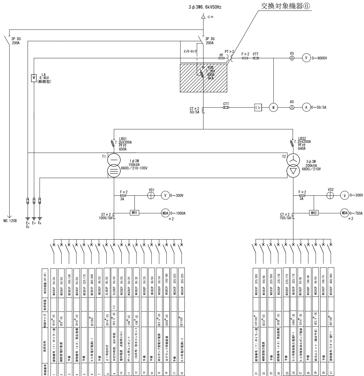
図6.1-単線結線図 (No.9)
