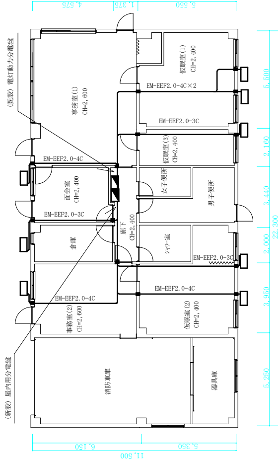
二次側電源配線平面図 S=1/150
