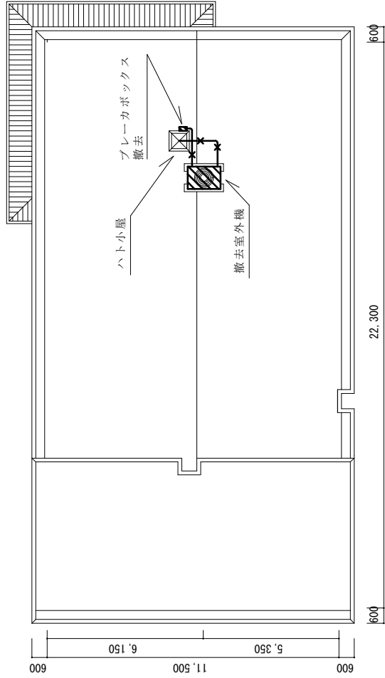
屋上撤去図 1/150
