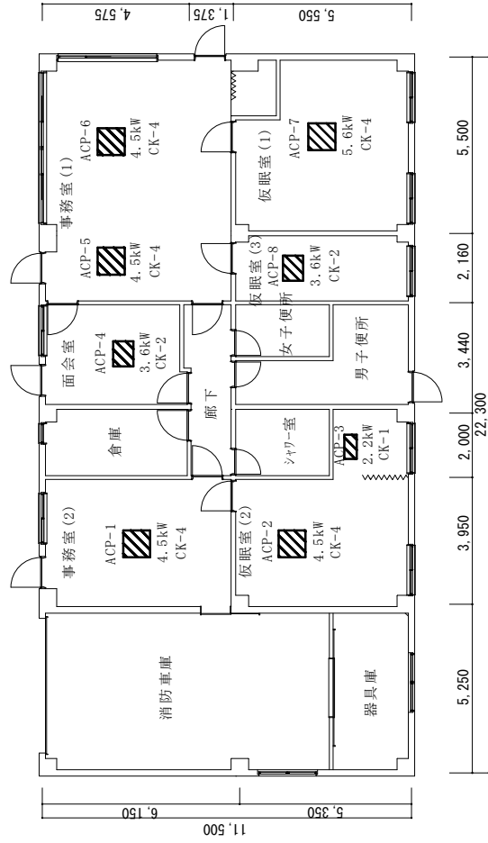
1 F 撤去図 1/150
