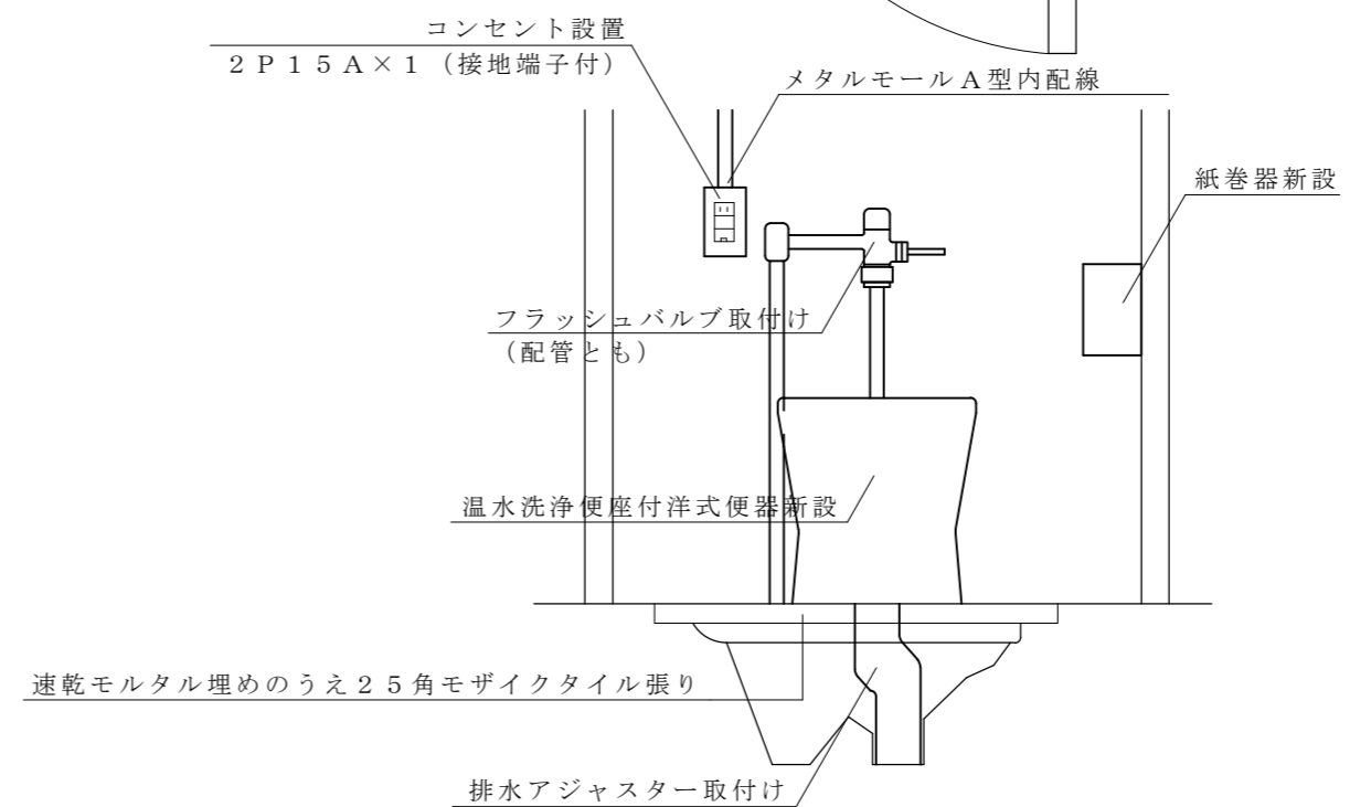
交換後断面図 S=1:15
