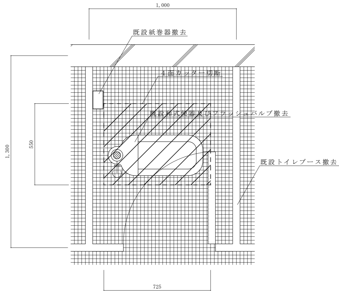
交換前平面図 S=1:15
