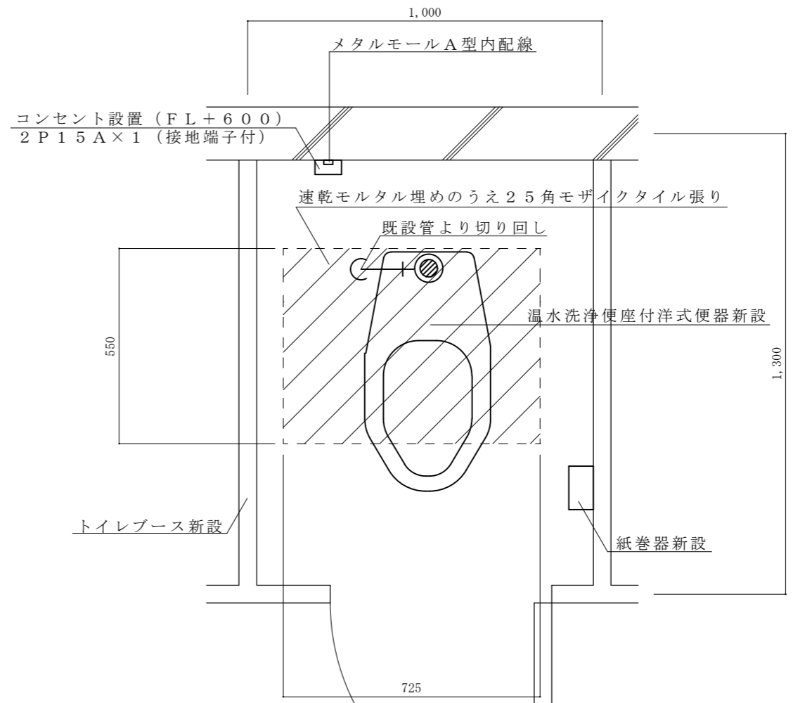
交換後平面図 S=1:15
