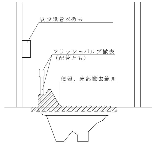
交換前断面図 S=1:15
