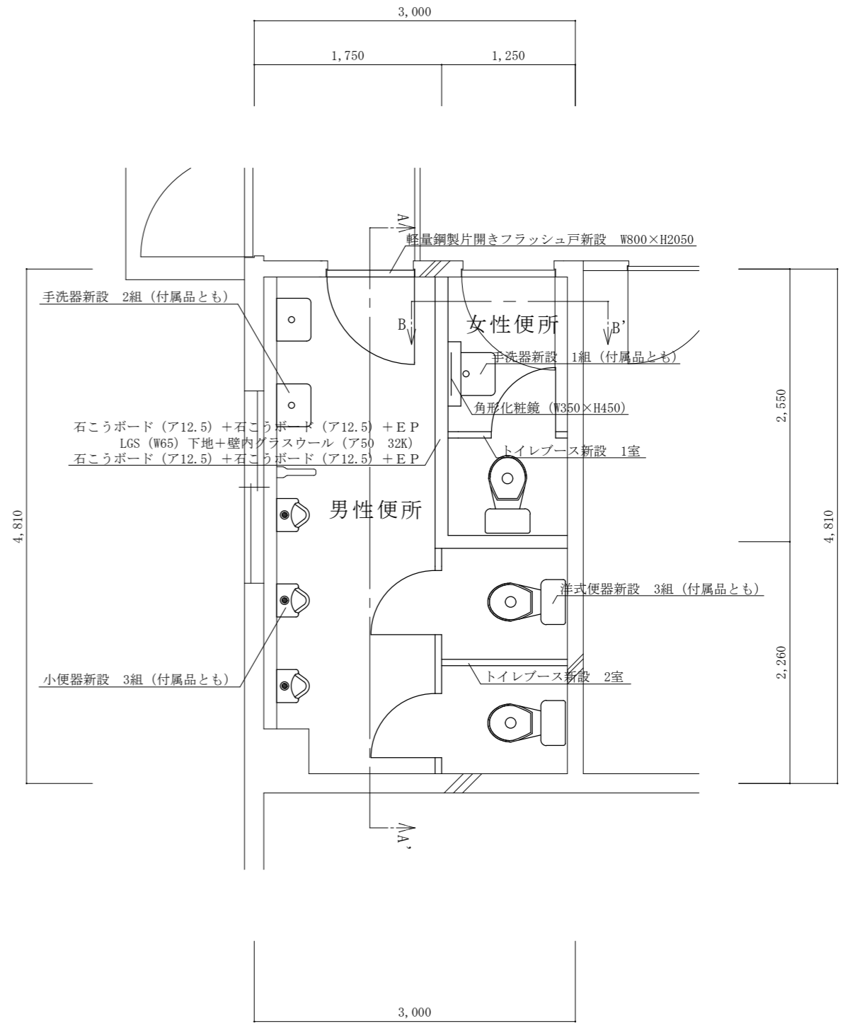
改修後平面図 S=1:50
