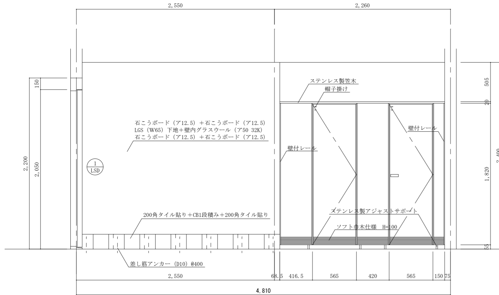
A - A' 断面図 S=1 : 30
