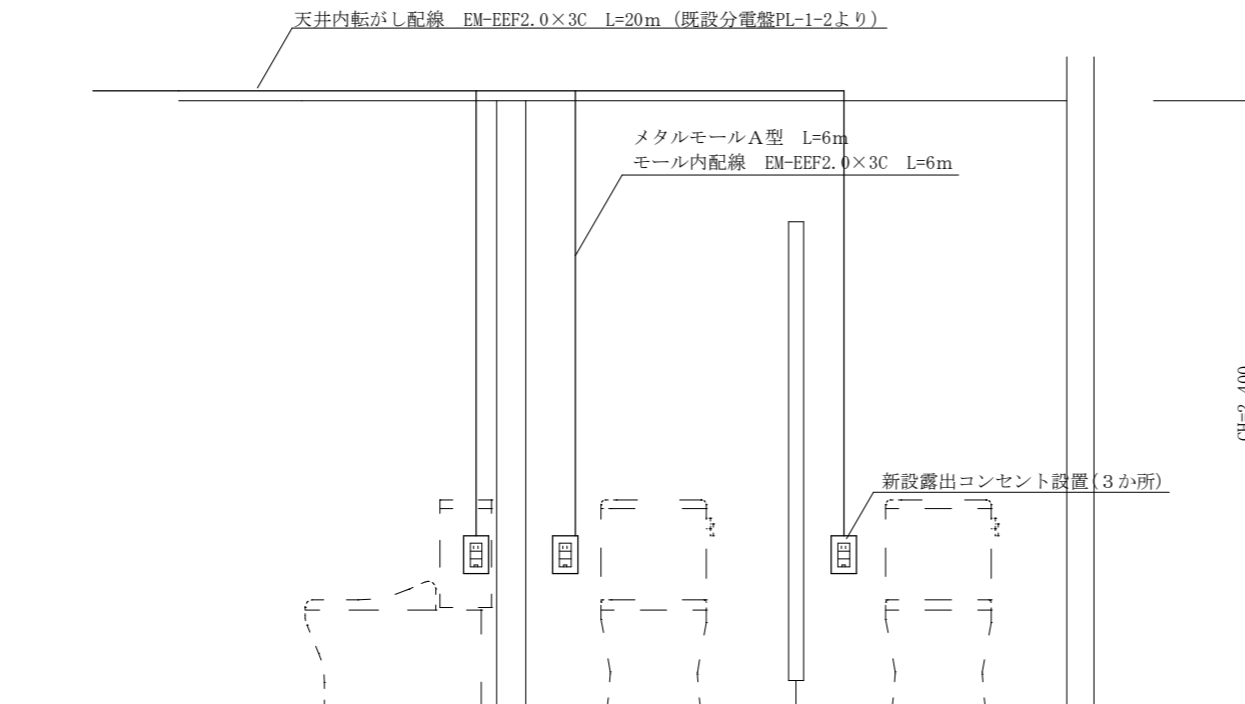
便所内コンセント配線図 S=1:30
