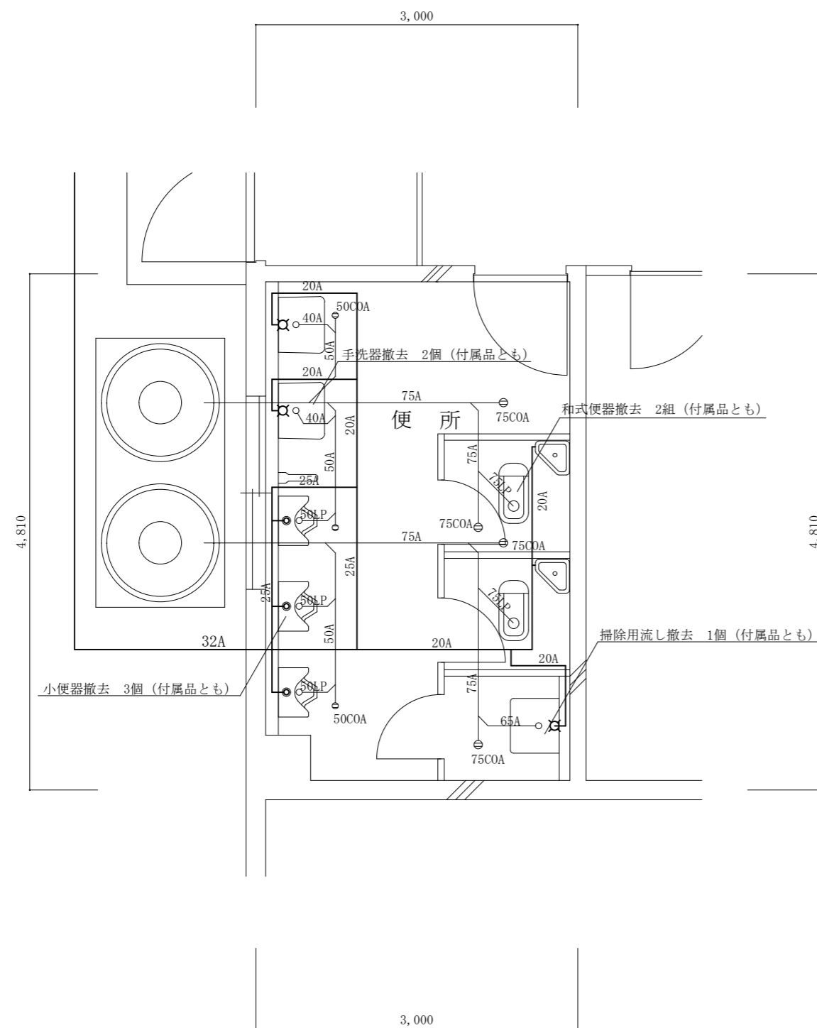
改修前給排水配管図 S=1:50
