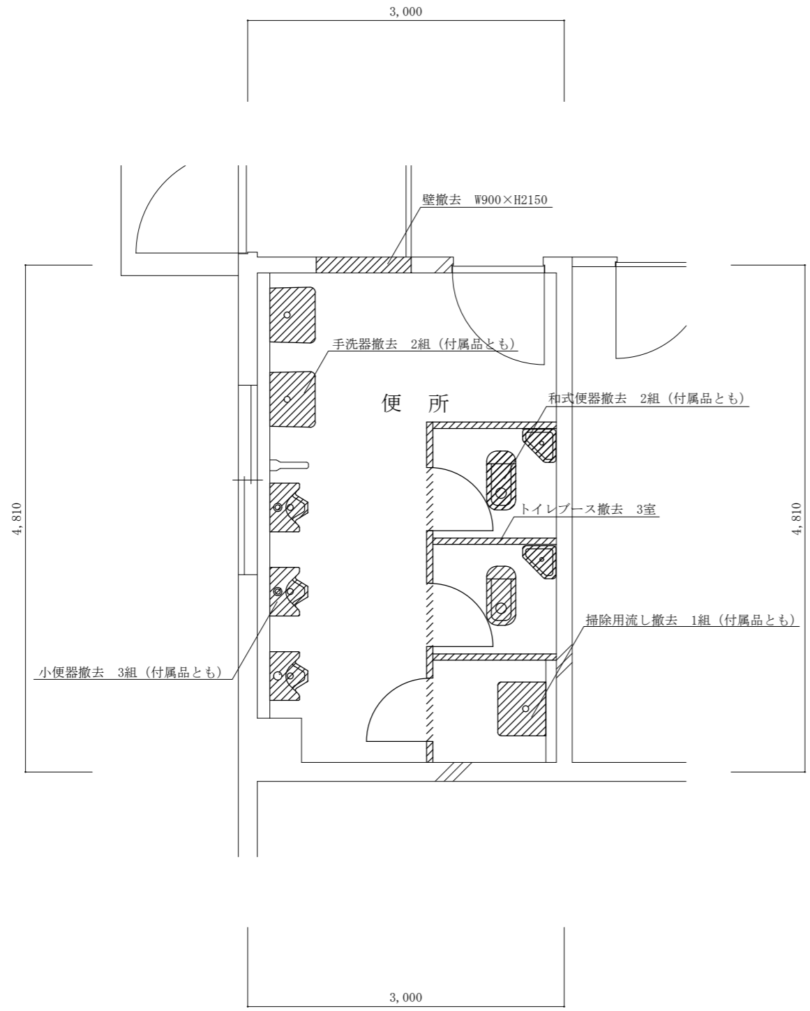
改修前平面図 S=1:50
