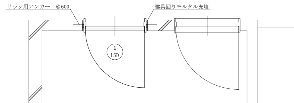
改修後建具回り詳細図 S=1:30
