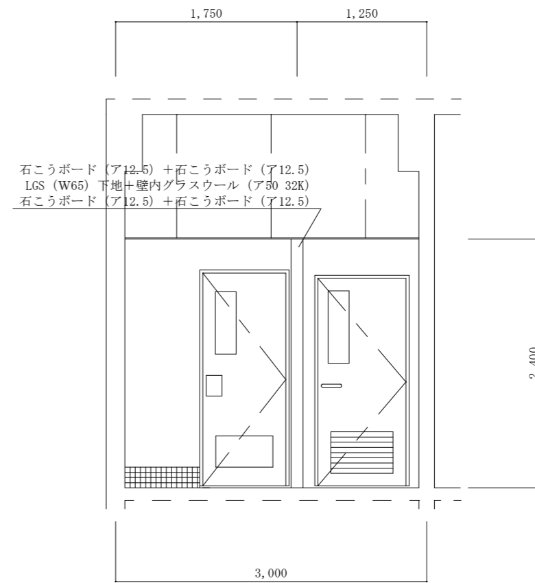
改修後断面図 S=1:50
