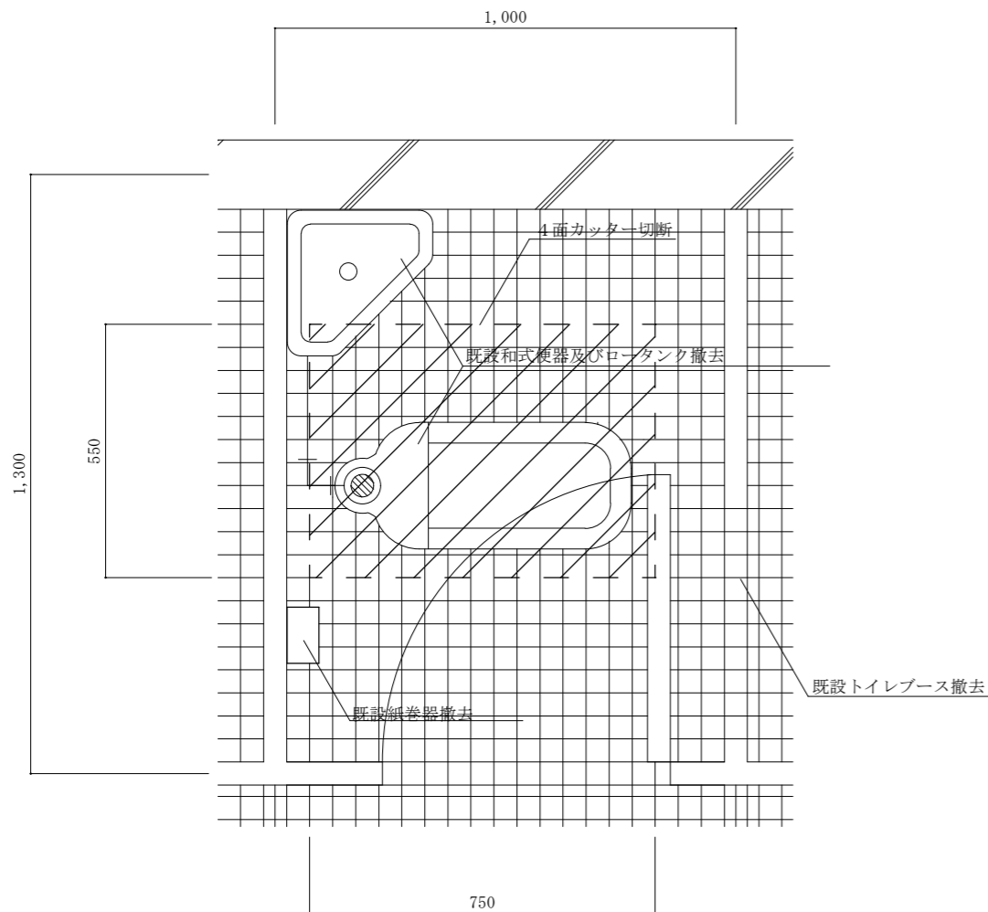
交換前平面図 S=1:15
