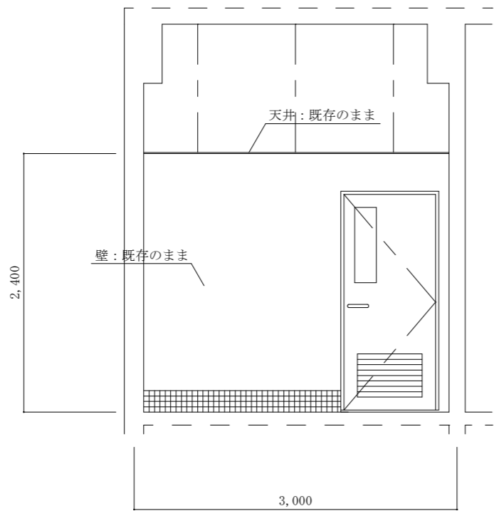
改修前断面図 S=1:50
