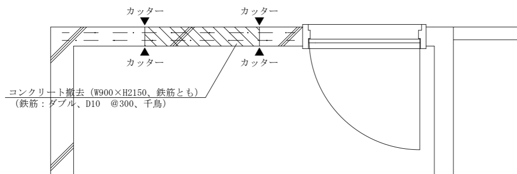
改修前建具回り詳細図 S=1:30
