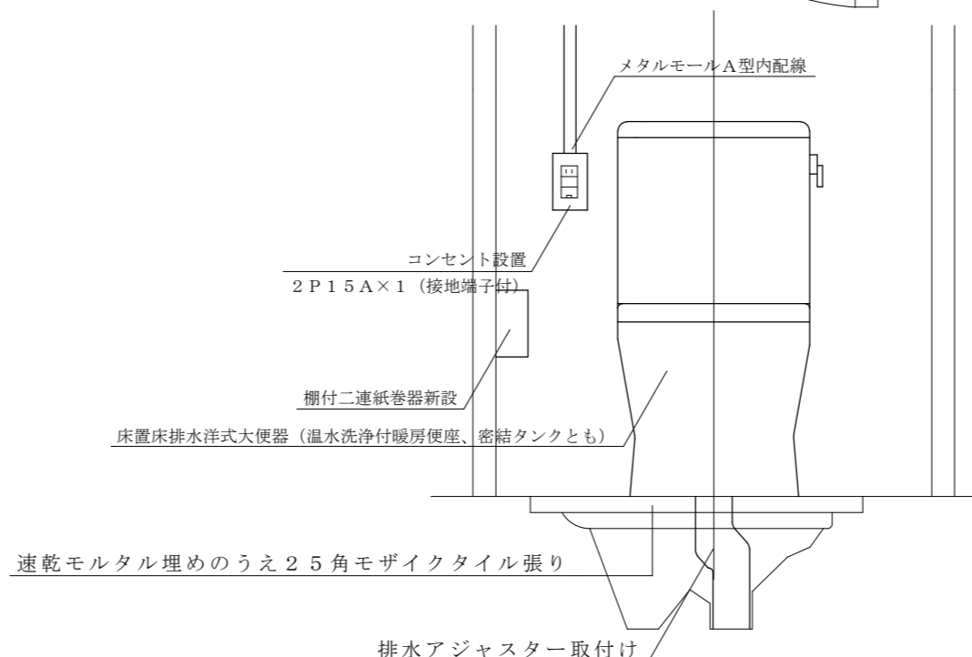
交換後断面図 S=1:15
