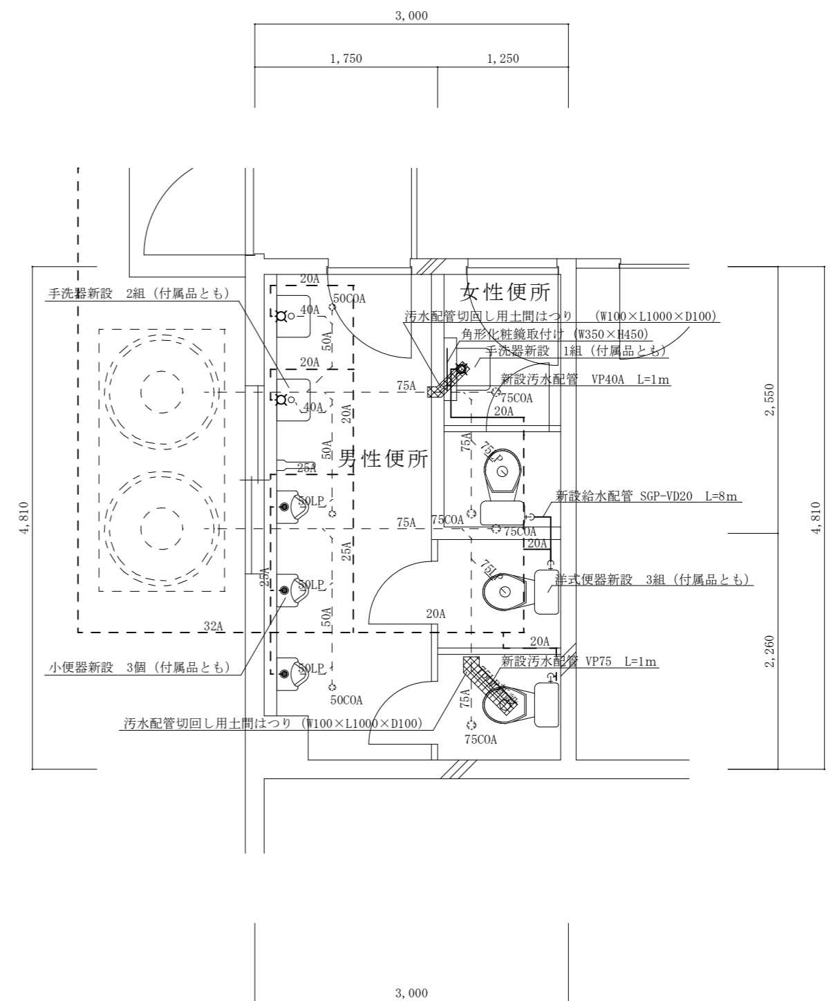
改修後給排水配管図 S=1:50
