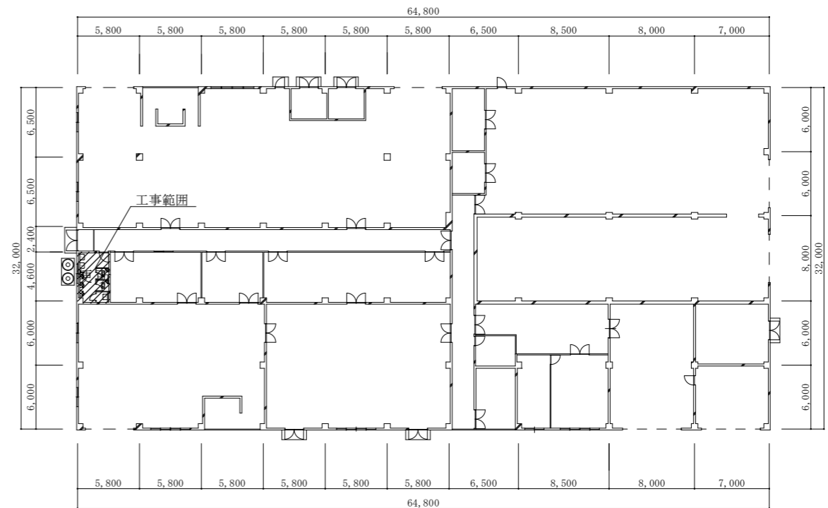
平面図 S=1:500
