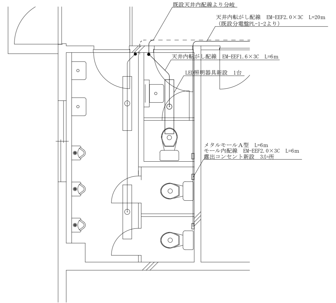
改修後電気配線図 S=1:50
