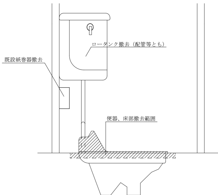
交換前断面図 S=1:15
