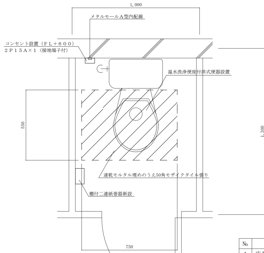
交換後平面図 S=1:15
