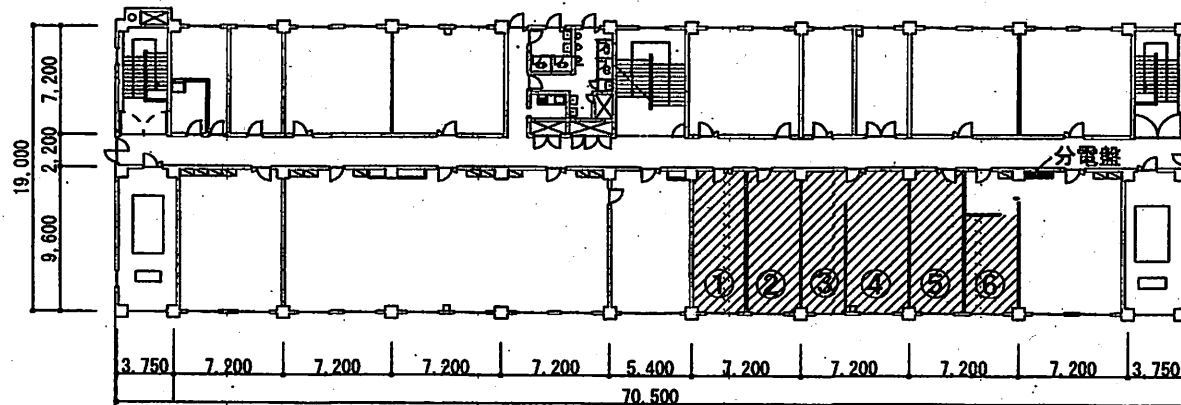
①第1庁舎 4階平面図 S=1:500
