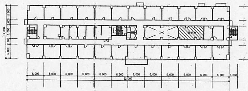
③第1隊舎2～7階平面図S=1:800
