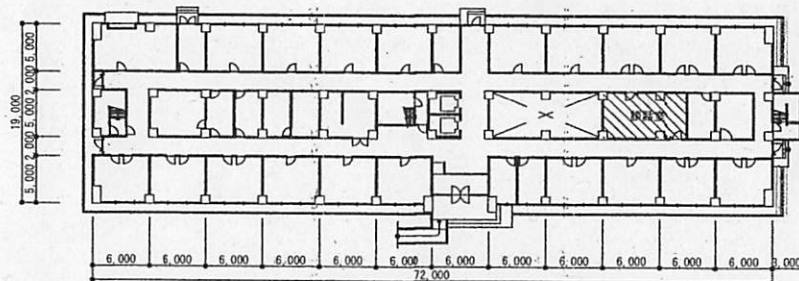
③第1隊舎1階平面図S=1:800
