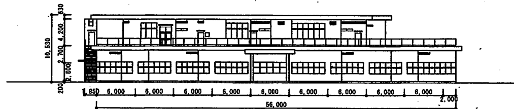
南立面図 S = 1 : 200
