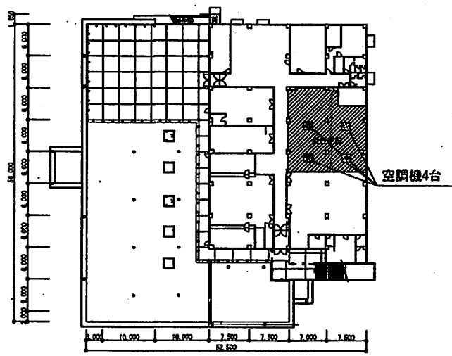
2階平面図 S = 1 : 200
