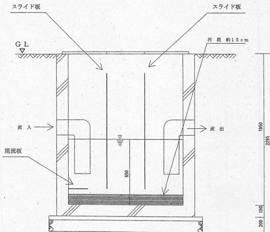
A-A断面図
