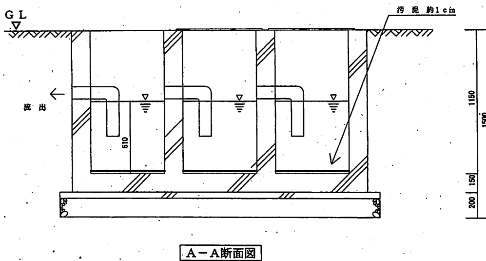
油分離槽（J-14庁舎燃料タンク）
