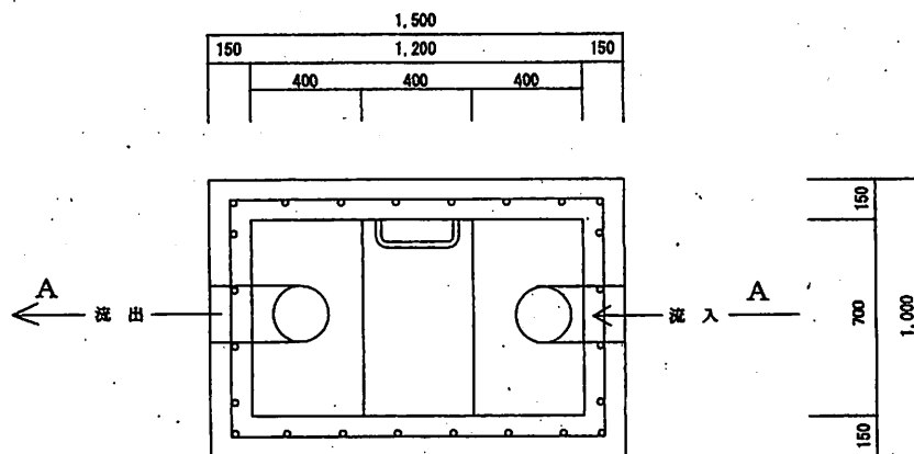
油分離槽平面図
