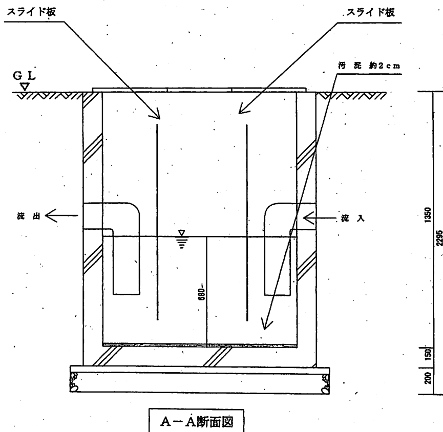
油分離槽 (J-22整備工場)
