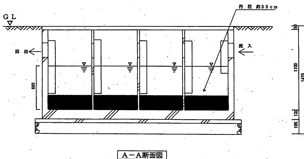
油分離槽 (洗車場)
