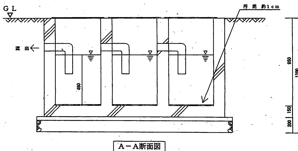
油分離槽（J-10予備電源室燃料タンク）
