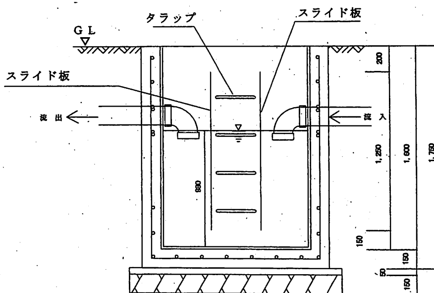
A-A断面図
