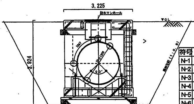
5KLタンク側面図 S=1:X
