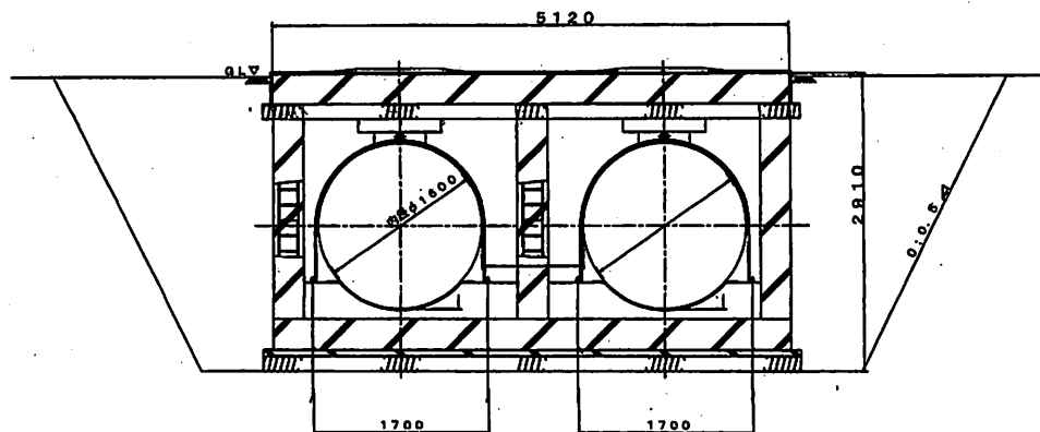
10KLタンク側面図 S=1:X
