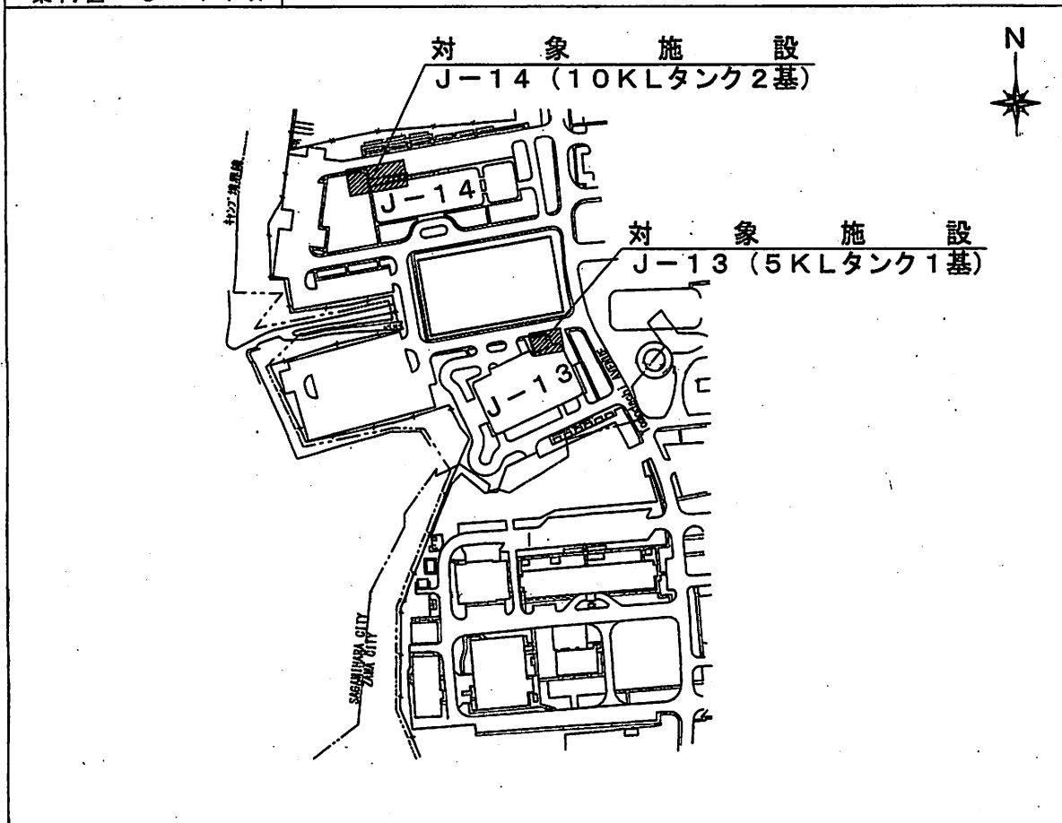
配置図 S = 1 : X
