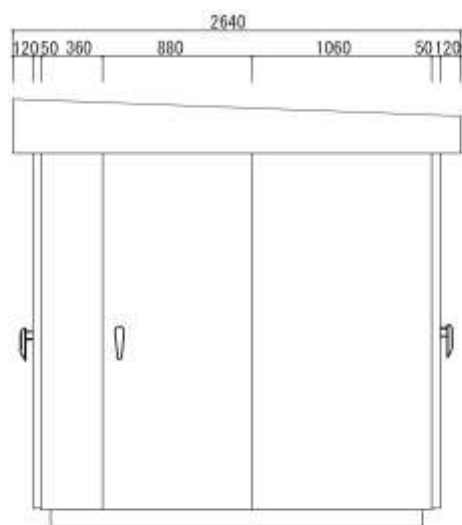
No. 1 キュービクル 正面図
