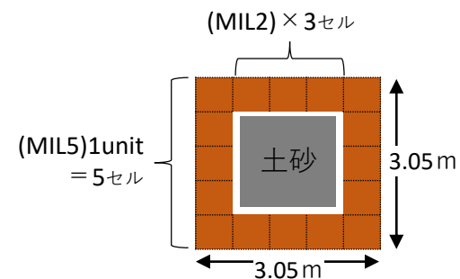
最上段平面図 (MIL5・MIL2)
