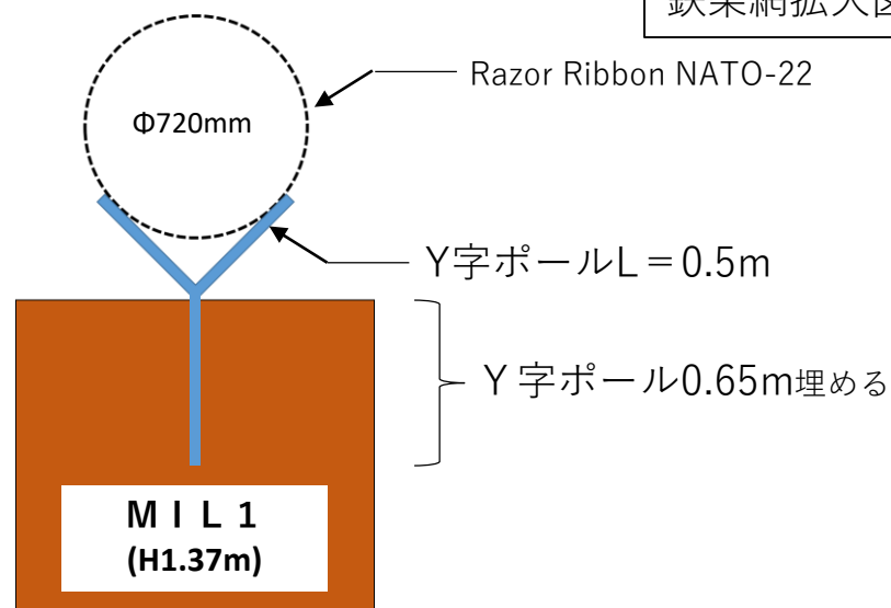
鉄条網拡大図
