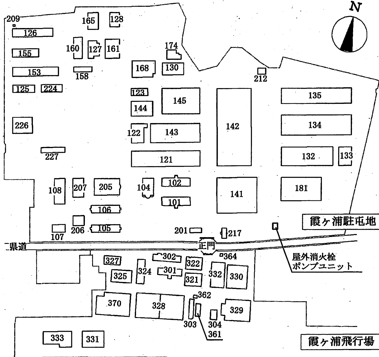
配置図 S=1/x
