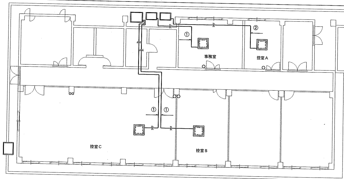
冷媒管平面図 S=1/200
