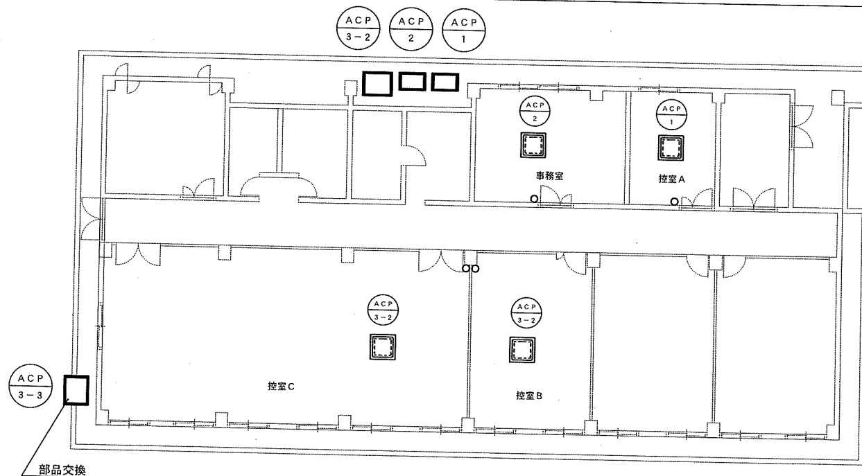
5号建物1F平面図 S=1/200
