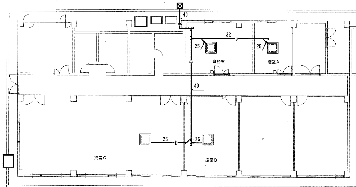
ドレン管平面図 S=1/200
