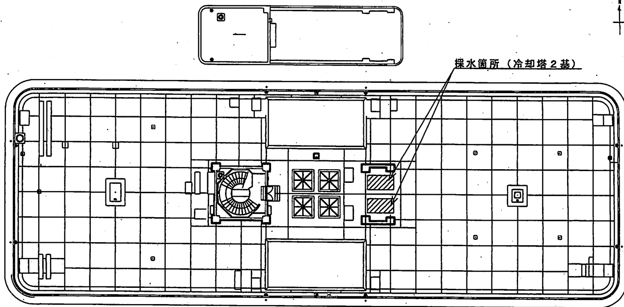
J-14庁舎RF S=1/X
