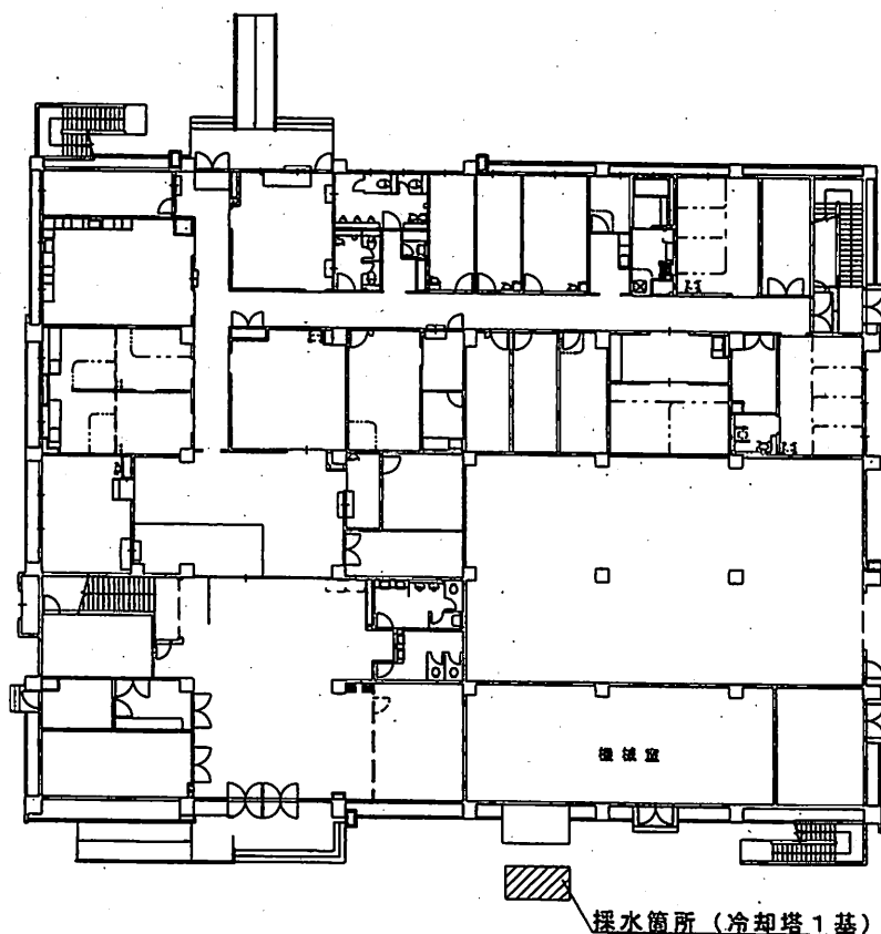
J-11厚生施設1F S=1/X
