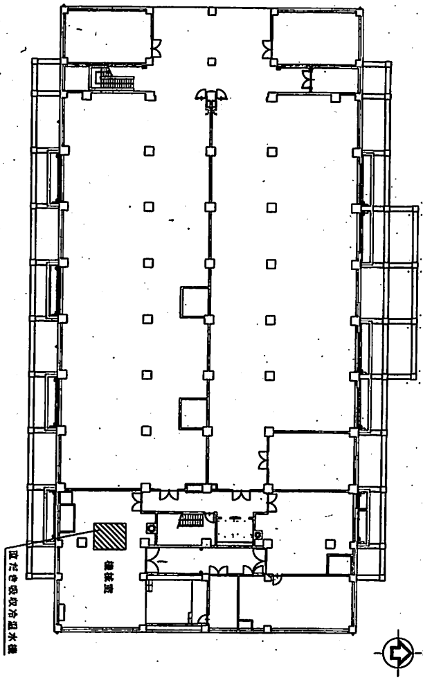
平面图 J-13 業務隊庁舎B1F S=1/X
