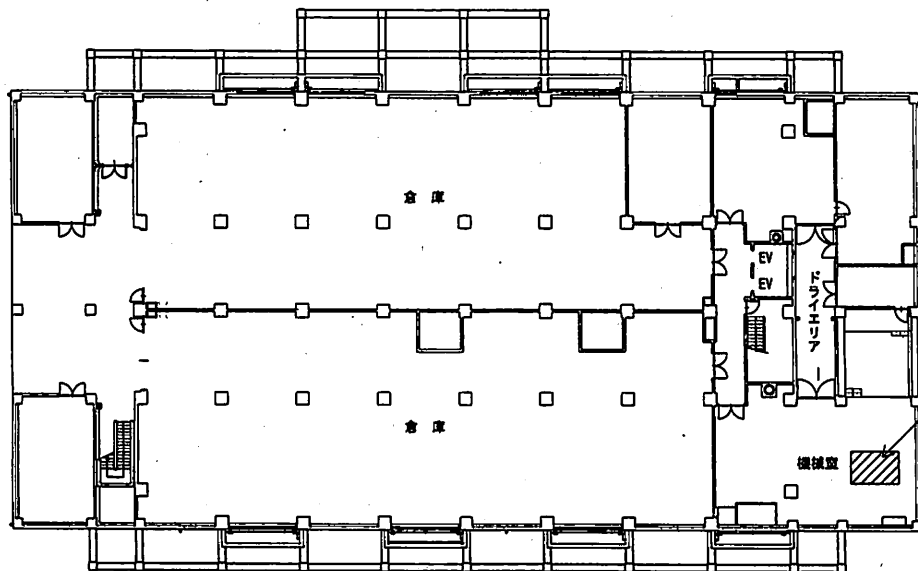
J-13 隊庁舎地下1階平面図 (S=1/500)
