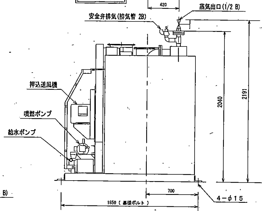
側面図
