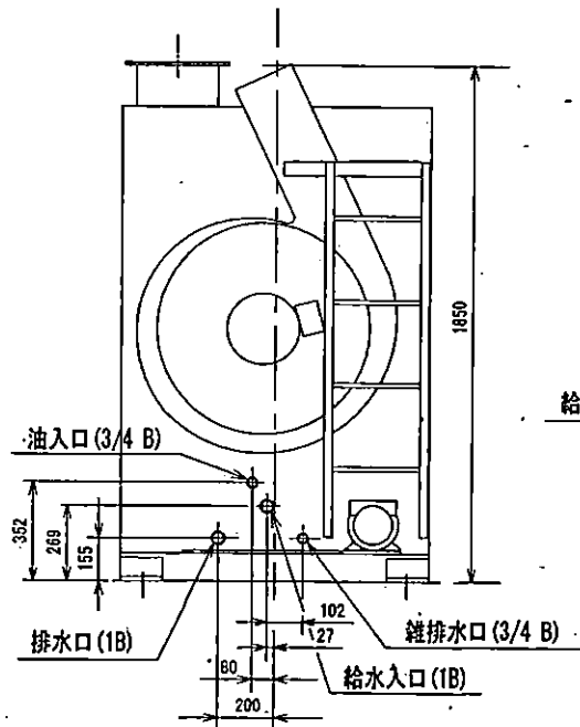
裏面図
