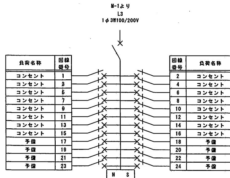
3L-1 壁掛型 (3階西側屋内)
