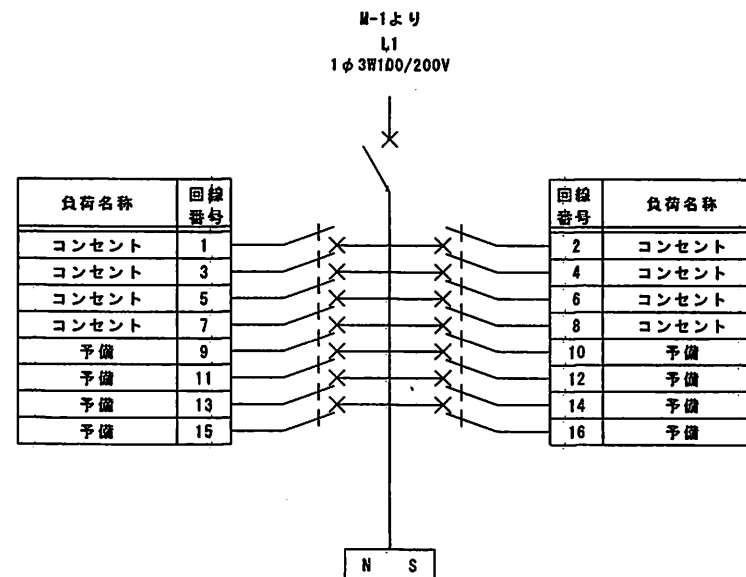
1L-1 壁掛型 (1階西側屋内)
