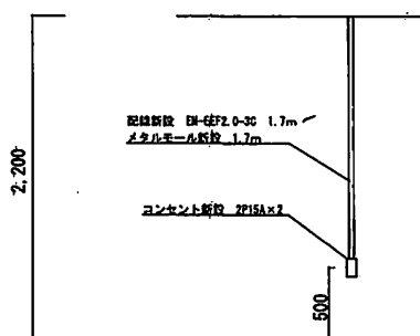
2号建物コンセント位置図 S=1/40
