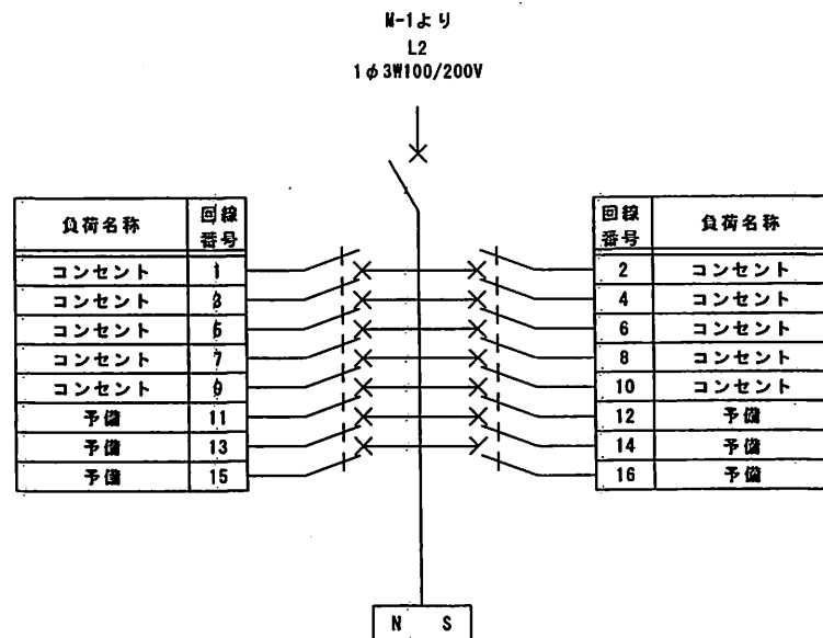
2L-1 壁掛型 (2階西側屋内)
