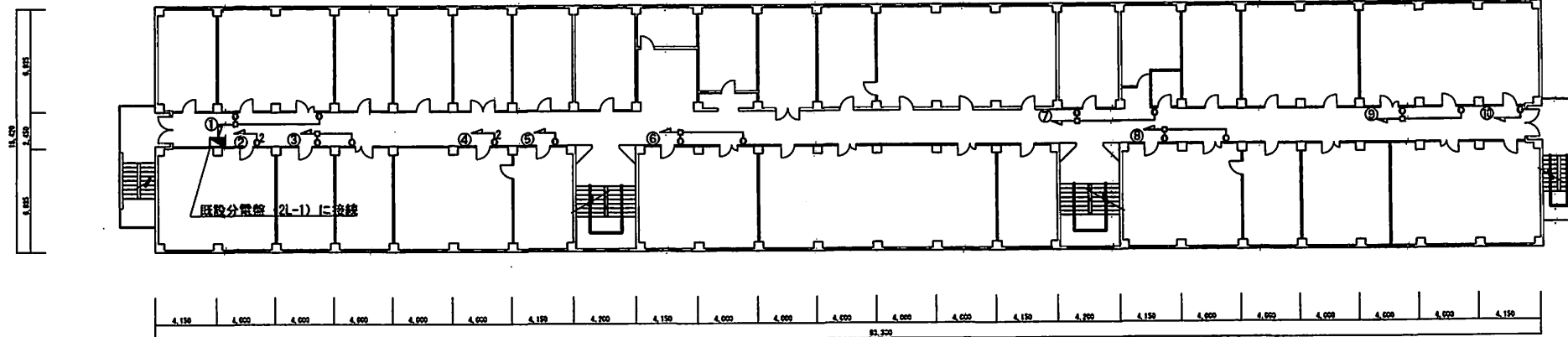
1号建物2階電灯設備図 S=1/300
