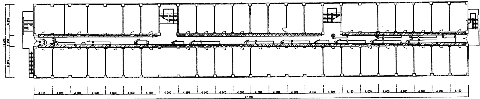
2号建物3階平面図 S=1/300
