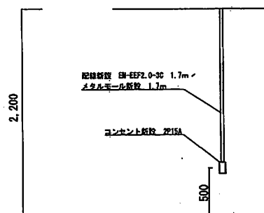
1号建物コンセント位置図 S=1/40
