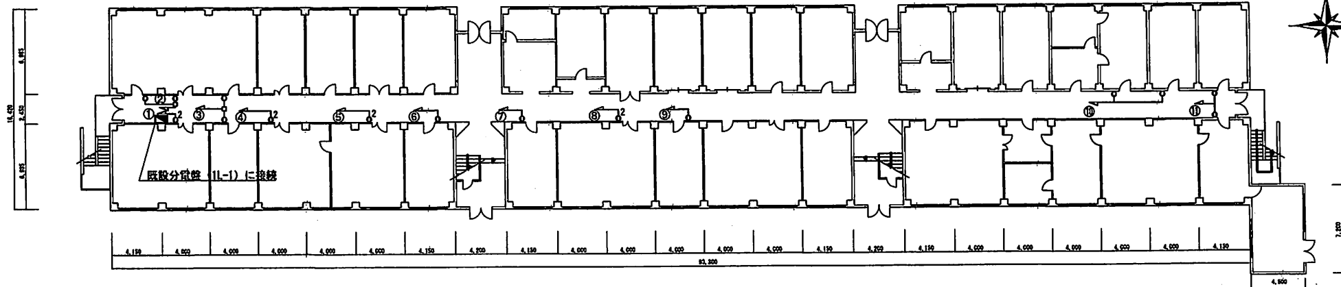
1号建物1階電灯設備図 S=1/300
