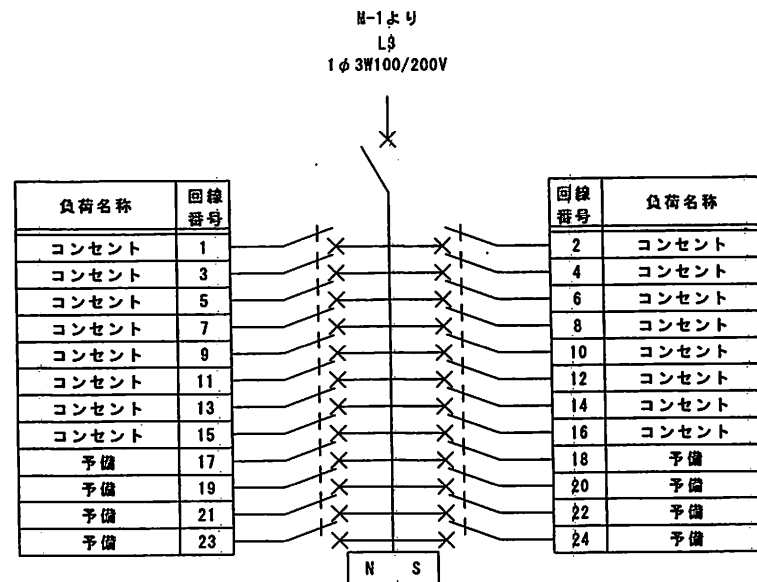
3L-1 壁掛型 (3階西側屋内)
