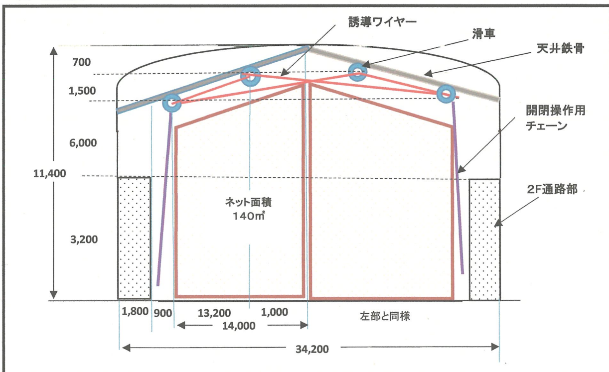
(2) 正面図
