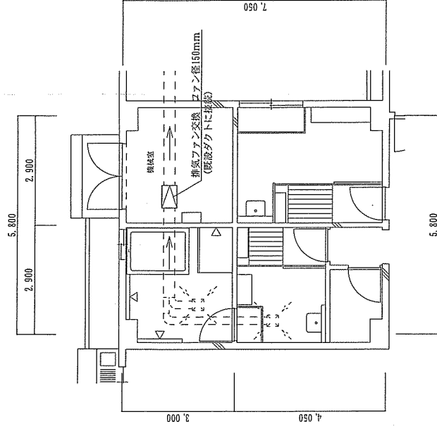
平面図 S=1:100
