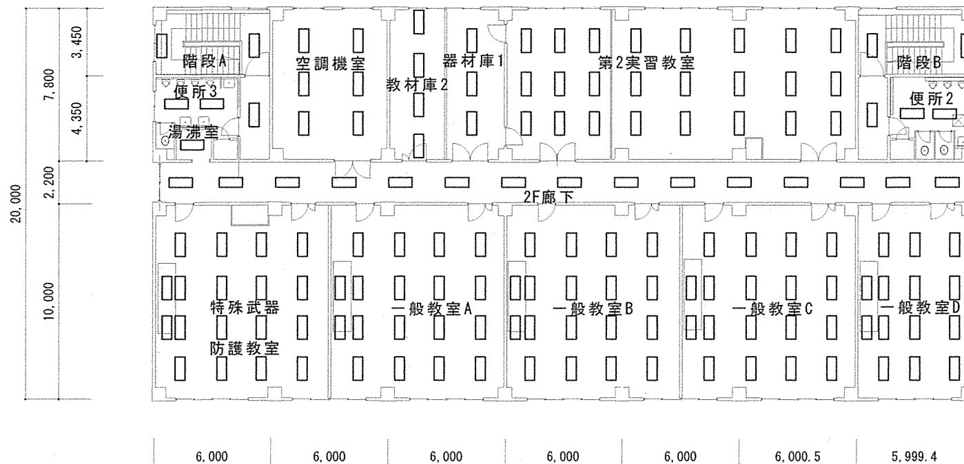
総合教場 2階平面図
