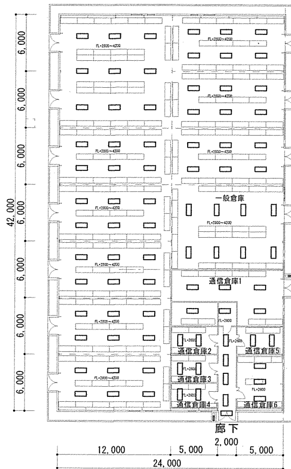
倉庫B 1階平面図
