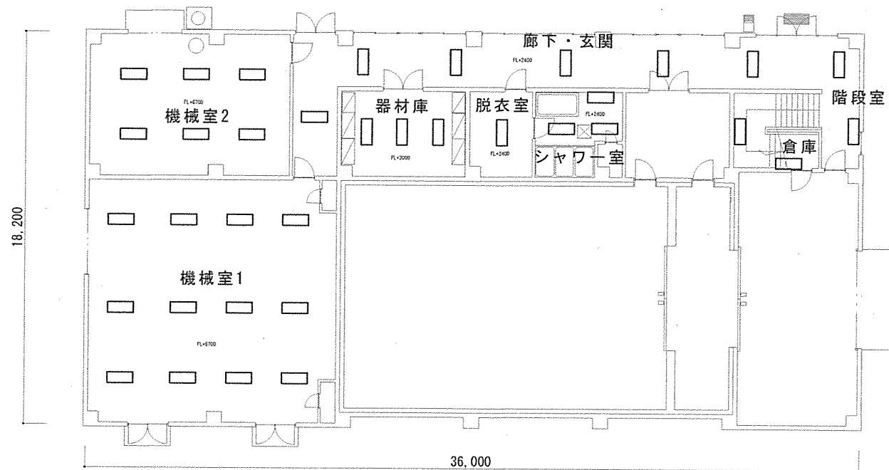
第2研究棟 1階平面図
