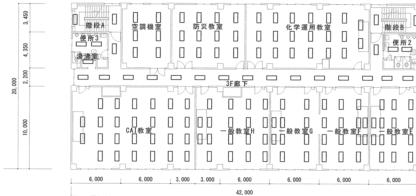
総合教場 3階平面図
