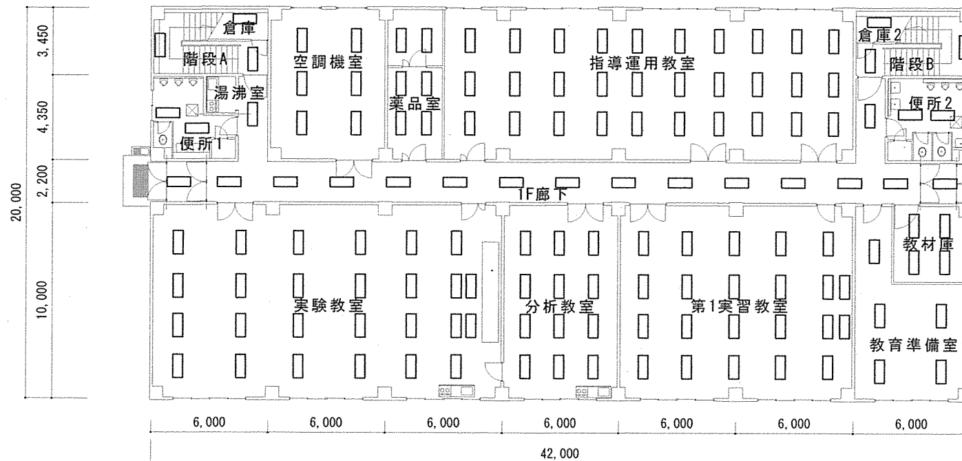
総合教場 1階平面図
