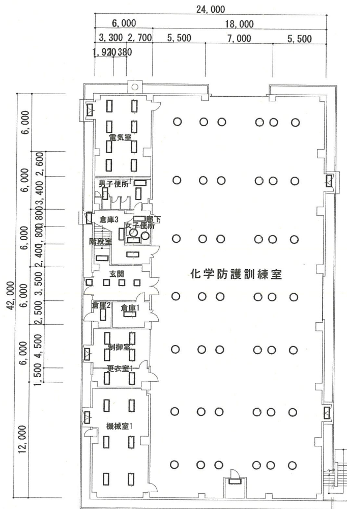
屋内訓練場 1階平面図
