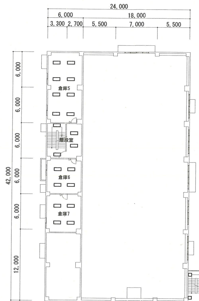
屋内訓練場 2階平面図
