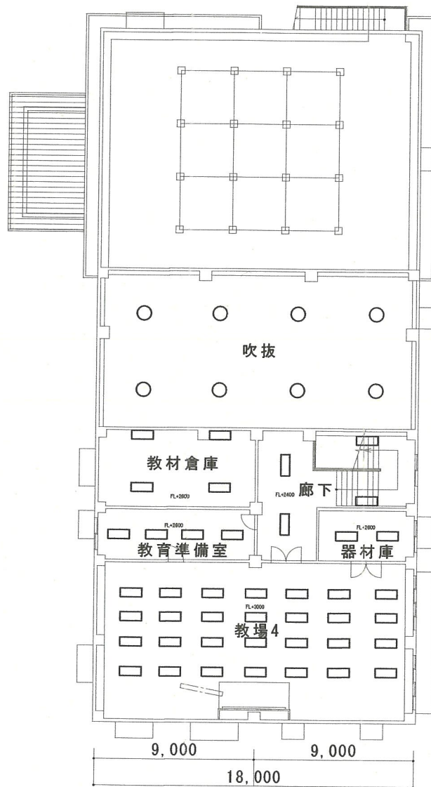
器材教場 2階平面図
