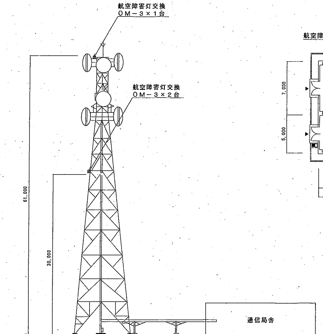
通信鉄塔姿図 S=1:Non
