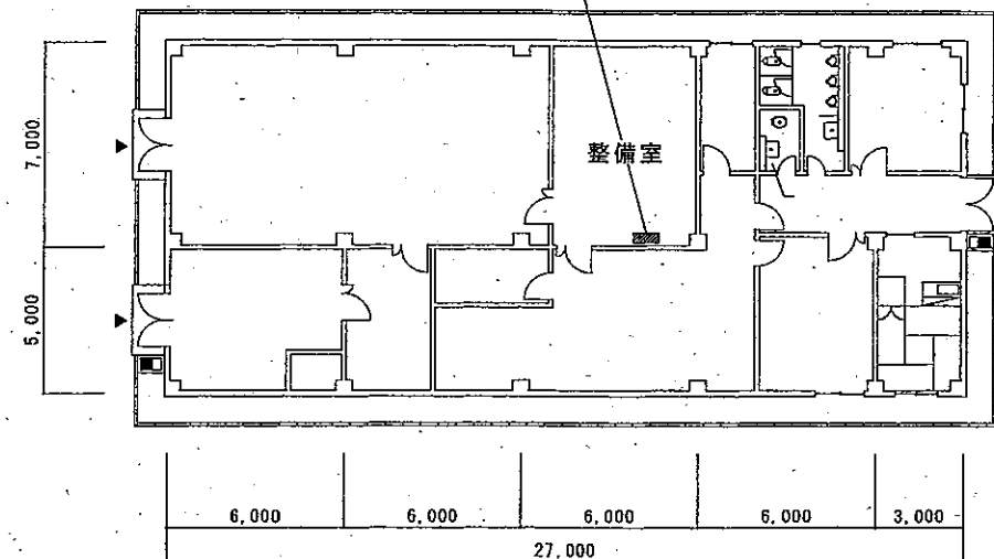
航空障害灯制御盤 (タイマーユニット)
